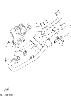
FIG. 10 ESCAPAMENTO
