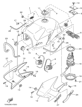
FIG. 25 TANQUE DE COMBUSTÍVEL P.34
