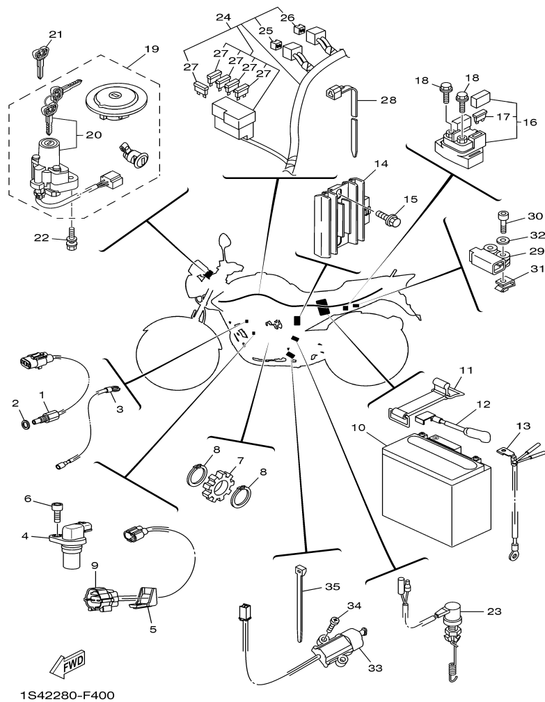
FIG. 40 SISTEMA ELÉTRICO 1
