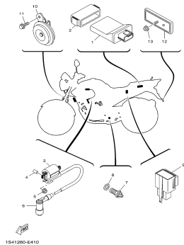
FIG. 41 SISTEMA ELÉTRICO 2
