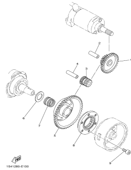
FIG. 13 EMBREAGEM DA PARTIDA
