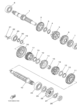
FIG. 15 TRANSMISSÃO
