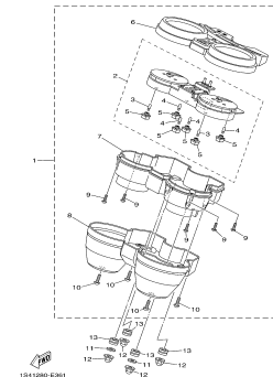
FIG. 36 MEDIDOR P.48
