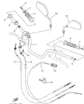
FIG. 30 GUIDÃO E CABOS P.41
