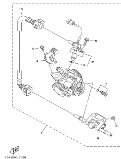
FIG. 9 ADMISSÃO 2
