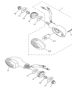
FIG. 35 PISCAS P.47
