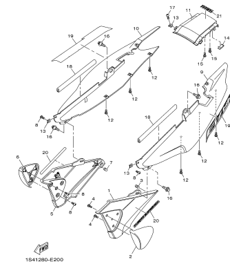
FIG. 20 TAMPA LATERAL
