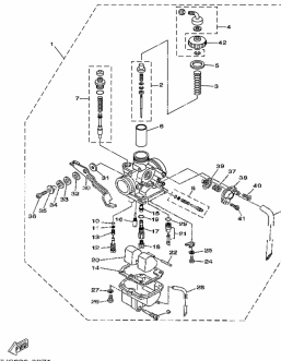
FIG. 7 CARBURADOR
