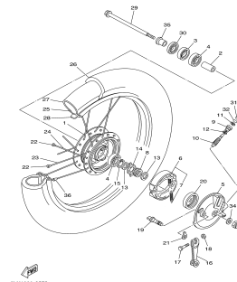
FIG. 24 RODA DIANTEIRA
