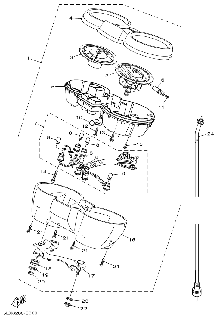
FIG. 30 MEDIDOR
