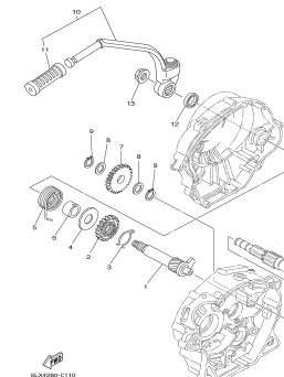
FIG. 11 PARTIDA
