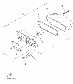
FIG. 32 LANTERNA TRASEIRA
