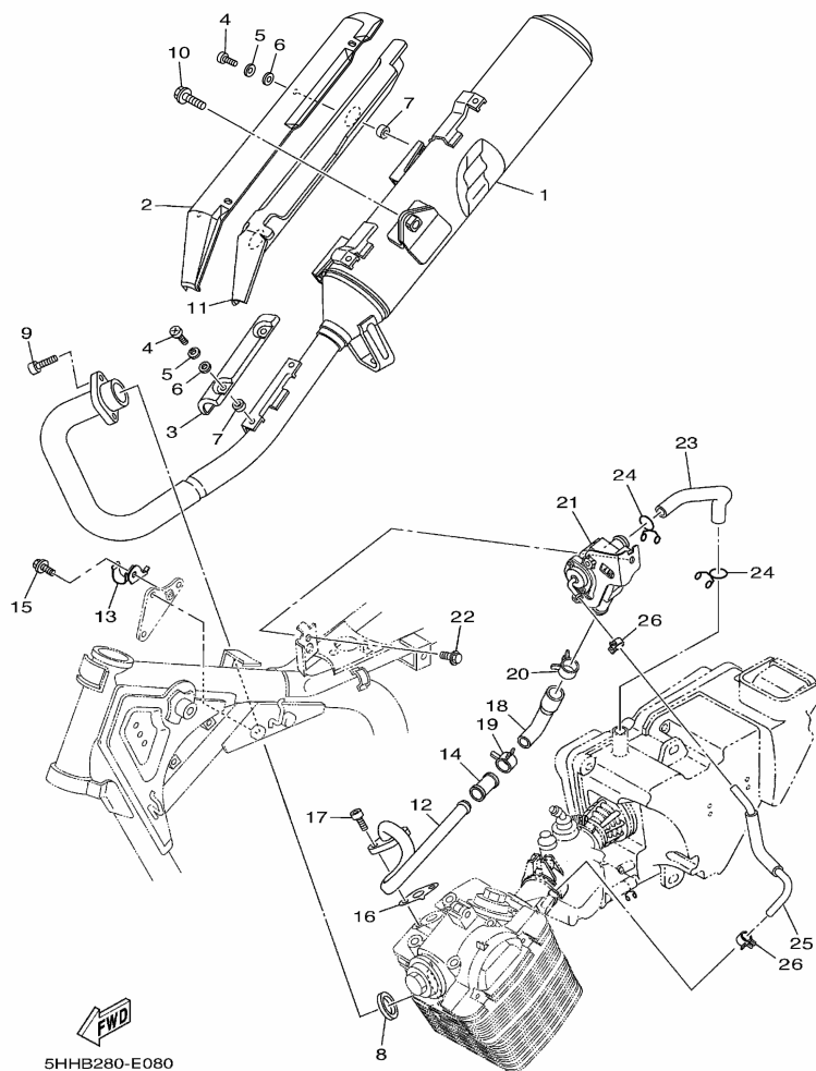
FIG. 8 ESCAPAMENTO
