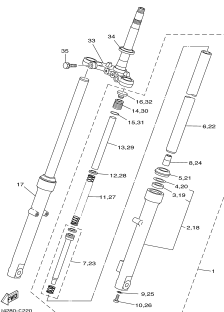
FIG. 21 GARFO DIANTEIRO
