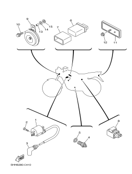
FIG. 35 SISTEMA ELÉTRICO 2
