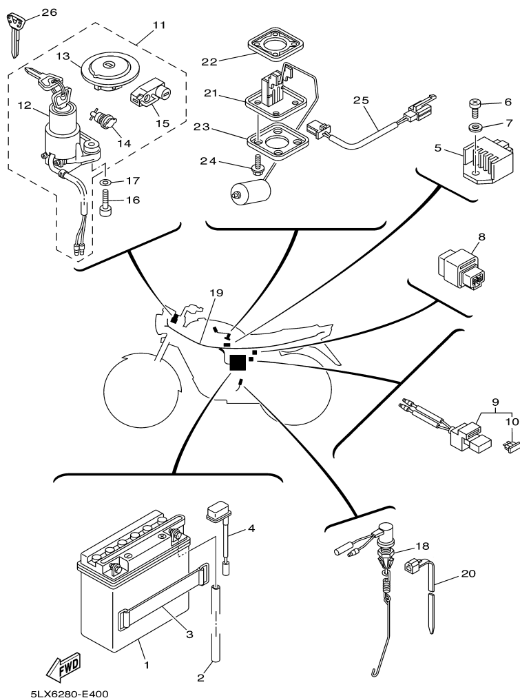
FIG. 34 SISTEMA ELÉTRICO 1
