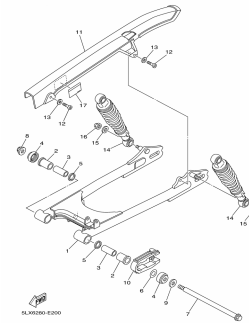
FIG. 19 GARFO TRASEIRO. SUSPENSÃO
