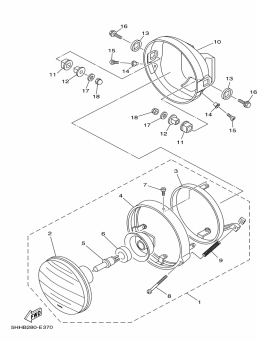
FIG. 31 FAROL DIANTEIRO
