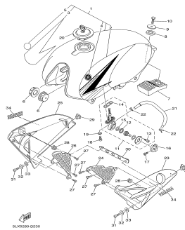
FIG. 22 TANQUE DE COMBUSTÍVEL
