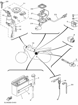
FIG. 34 SISTEMA ELÉTRICO 1
