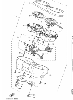
FIG. 30 MEDIDOR
