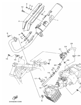
FIG. 8 ESCAPAMENTO
