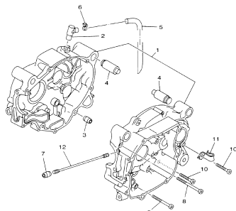
FIG.9 CARCAÇA DO MOTOR P.9
