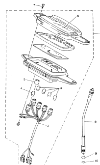
FIG.33 VELOCÍMETRO P.40
