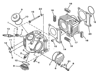
FIG.1 CABEÇOTE E CILINDRO P.1
