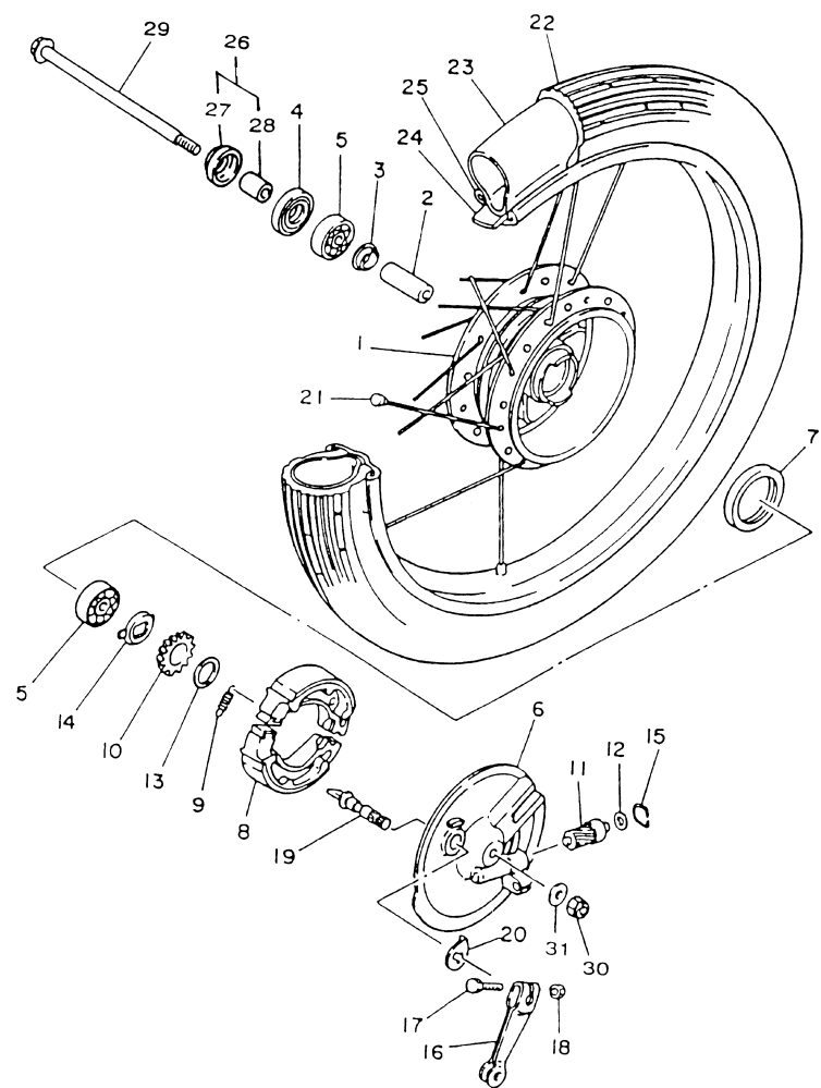
FIG. 25 - RODA DIANTEIRA
