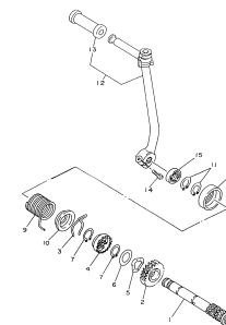
FIG.11 EIXO E PEDAL DE PARTIDA (OPCIONAL) P.11
