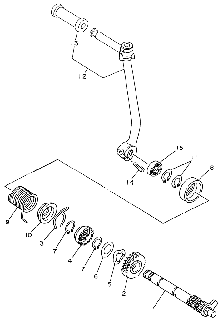
FIG. 11 - EIXO DE ARRANQUE
