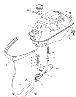
FIG.23 TANQUE DE COMBUSTÍVEL
