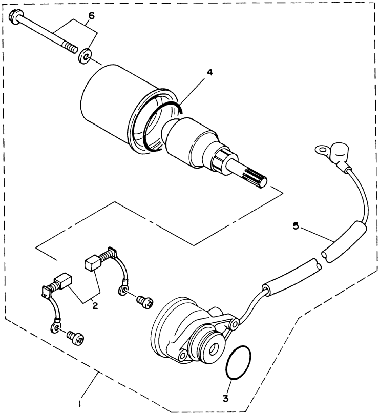
FIG. 31 - MOTOR DE PARTIDA
