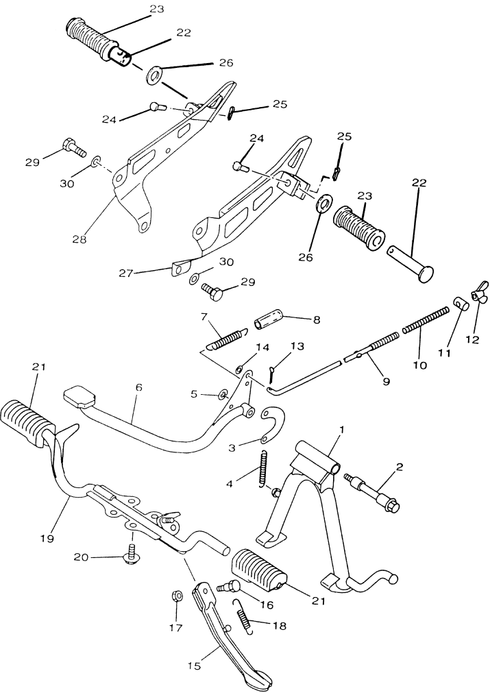
FIG. 28 - CAVALETE - ESTRIBOS E PEDAL DE FREIO
