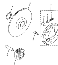
FIG.12 EMBREAGEM DA PARTIDA P.12
