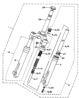
FIG.22 SUSPENSÃO DIANTEIRA
