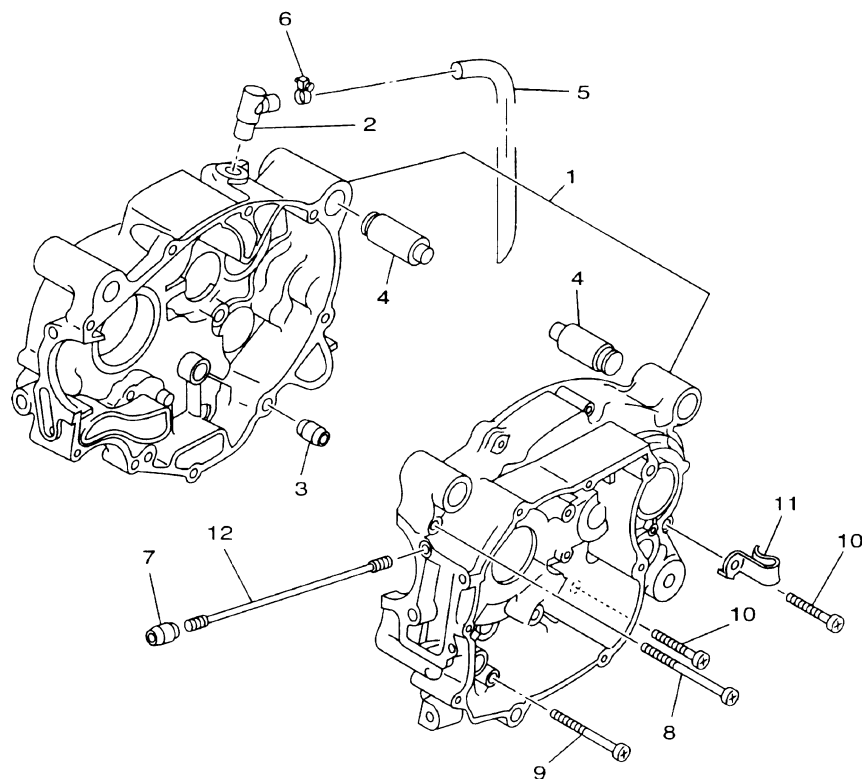
FIG. 09 - CARCAÇA DO MOTOR
