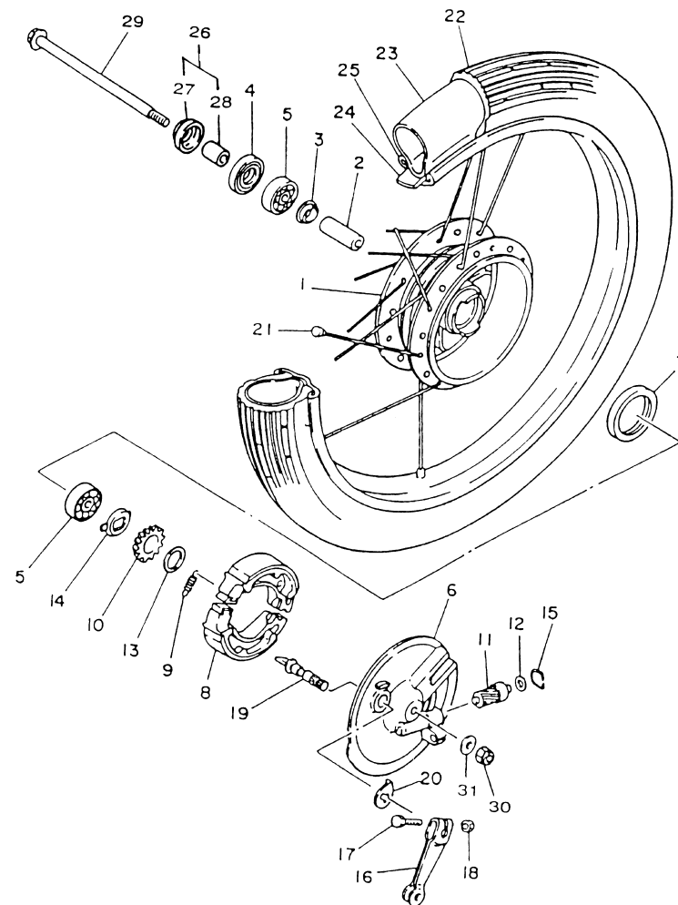
FIG. 25 - RODA DIANTEIRA
