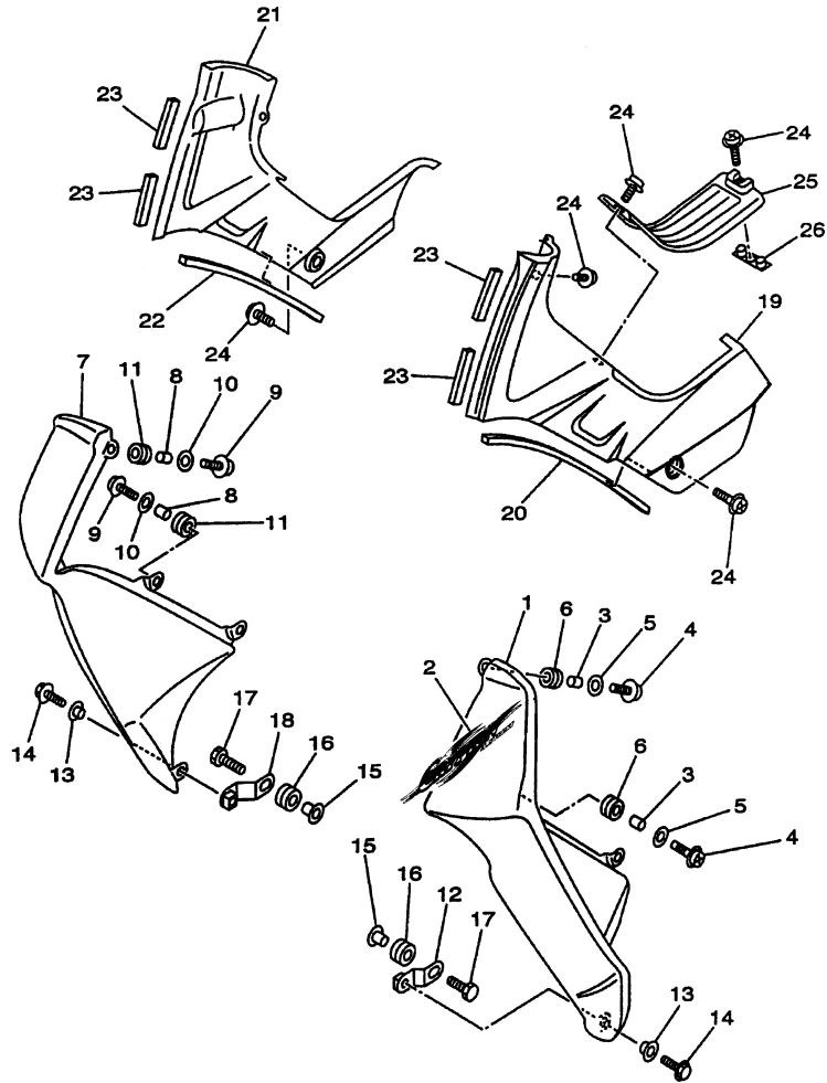
FIG. 29 - TAMPAS DIANTEIRAS
