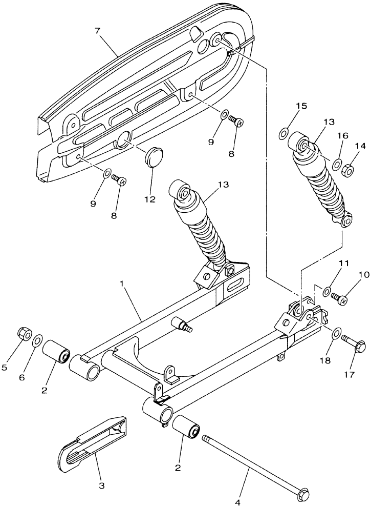
FIG. 20 - GARFO TRASEIRO
