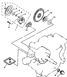
FIG.5 BOMBA DE ÓLEO P.5
