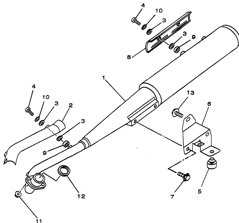
FIG. 08 - ESCAPAMENTO
