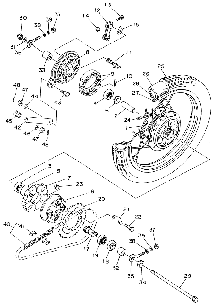
FIG. 26 - RODA TRASEIRA
