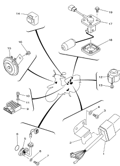
FIG.38 SISTEMA ELÉTRICO 2 P.45
