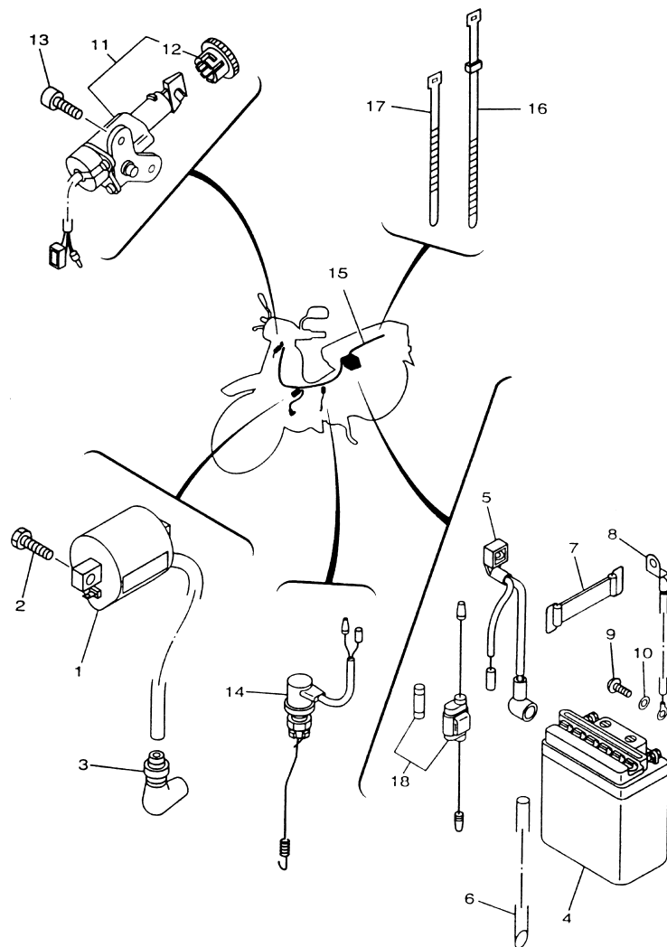
FIG. 37 - SISTEMA ELÉTRICO 1
