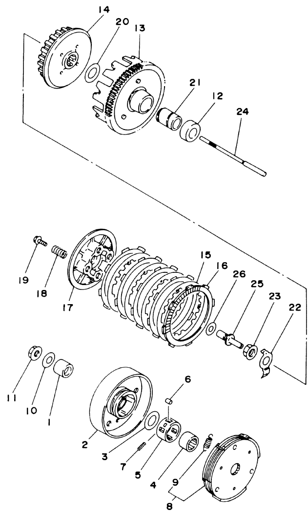
FIG. 13 - FRICÇÃO
