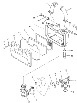
FIG.10 TAMPA DA CARCAÇA P.10
