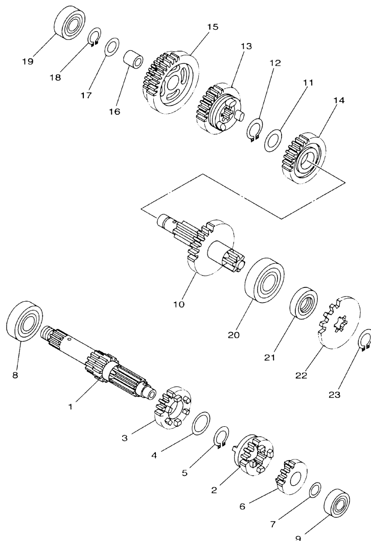
FIG. 14 - TRANSMISSÃO
