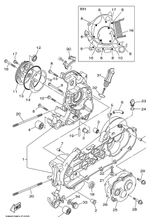
FIG. 10 CARÇA DO MOTOR
