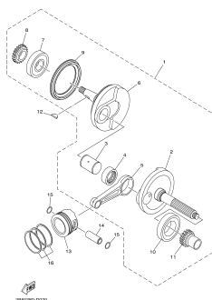
FIG. 2 VIRABREQUIM E PISTÃO
