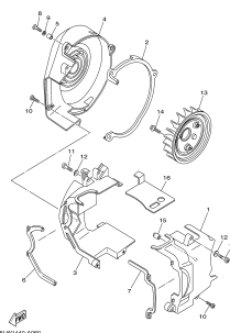
FIG. 10 CARÇA DO MOTOR
