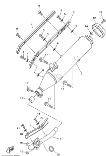
FIG. 9 ESCAPAMENTO
