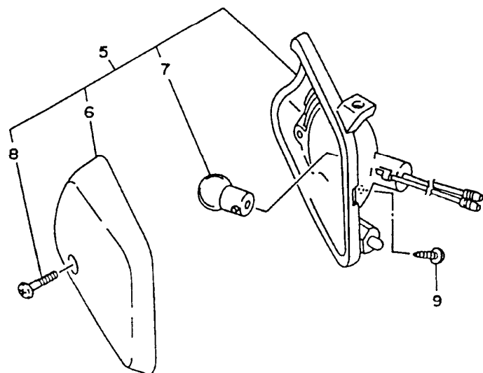
FIG. 32 - SINALIZADORES DIANTEIROS (PISCA-PISCA)
