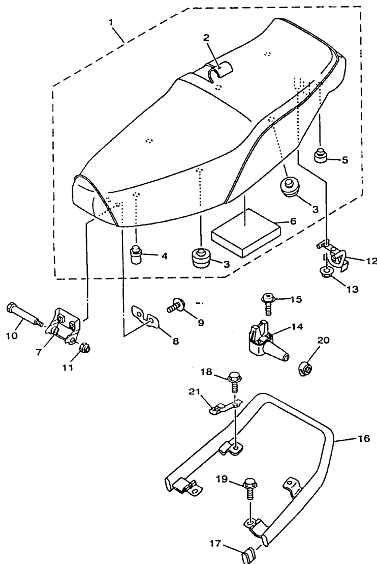
FIG. 24 - ASSENTO
