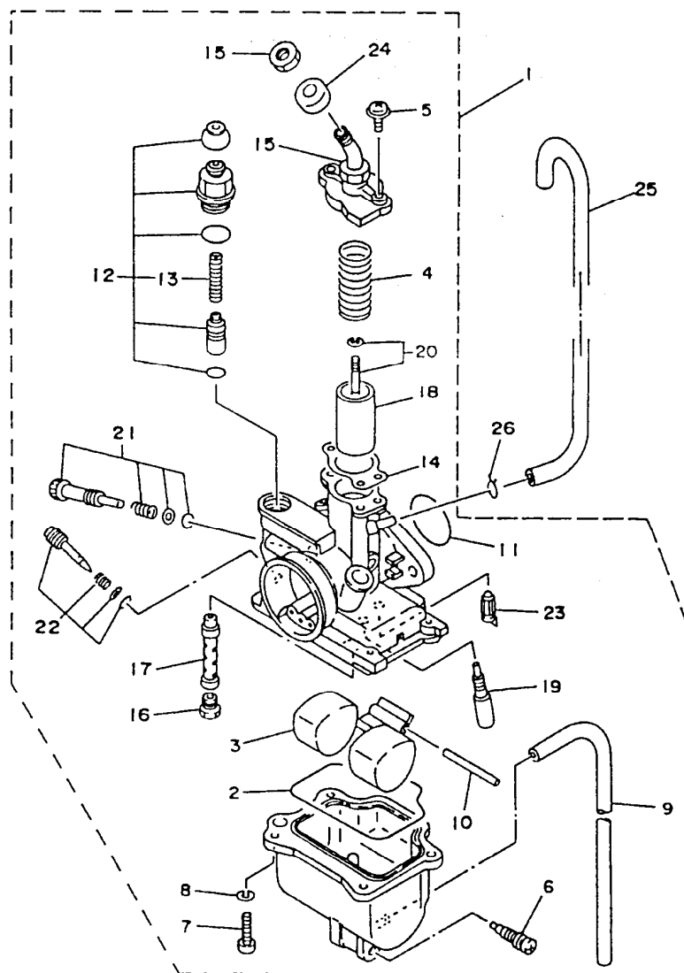
FIG. 07 - CARBURADOR
