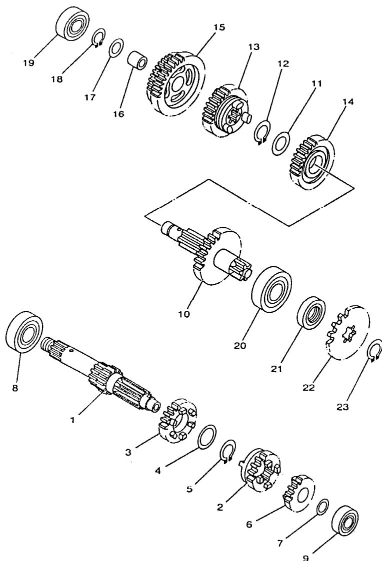
FIG. 14 - TRANSMISSÃO
