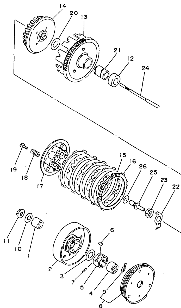
FIG. 13 - FRICÇÃO
