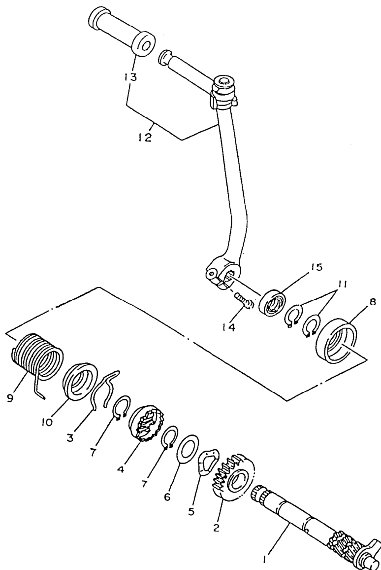
FIG. 11 - EIXO DE MUDANÇA
