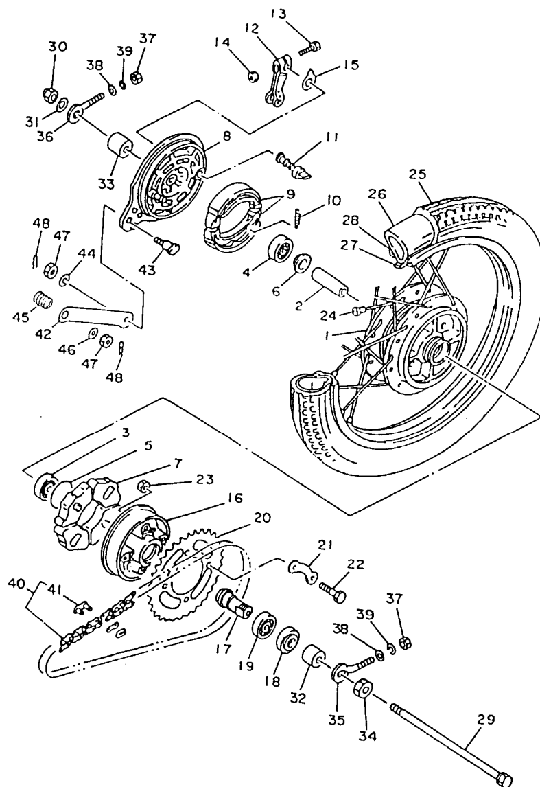
FIG. 26 - RODA TRASEIRA
