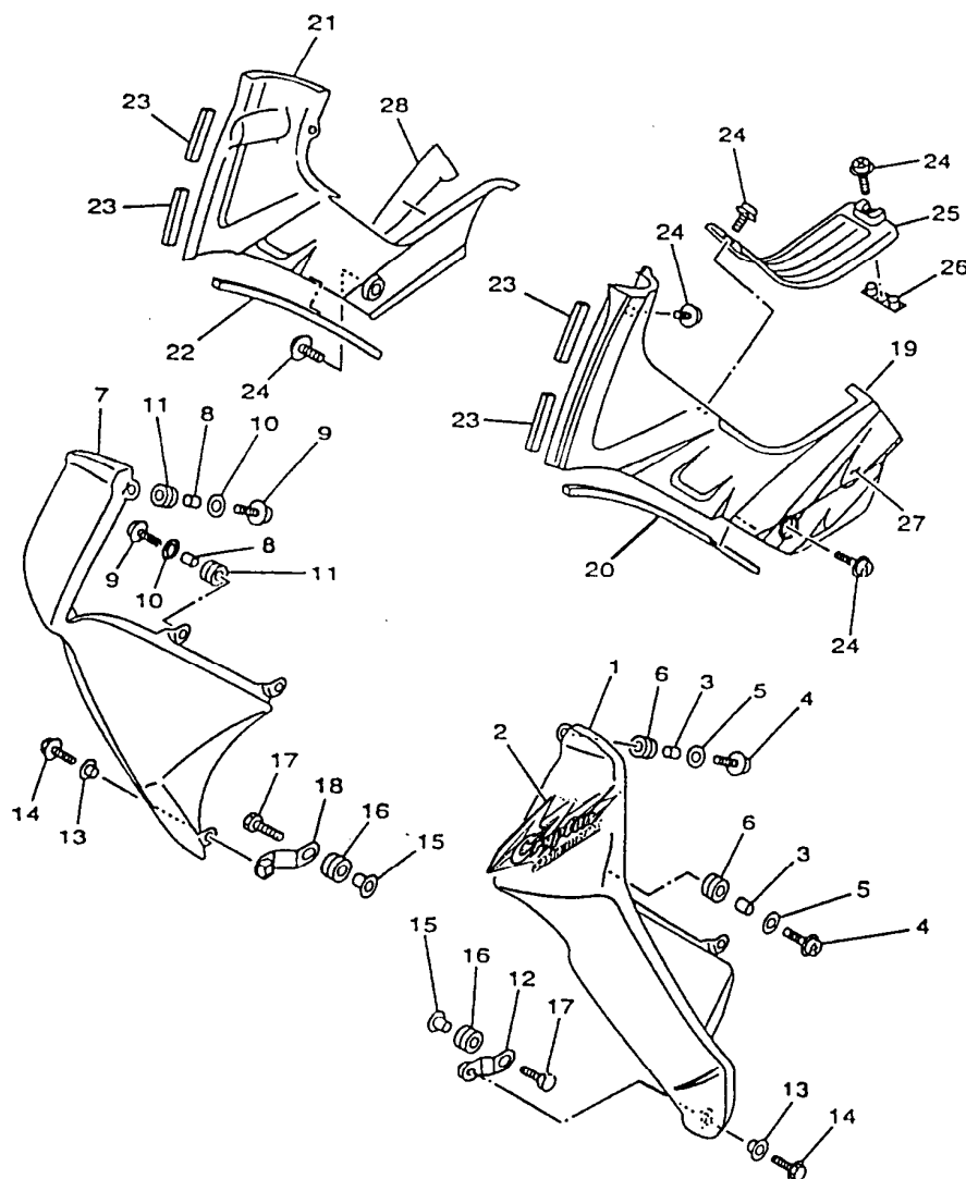
FIG. 29 - TAMPAS DIANTEIRAS
