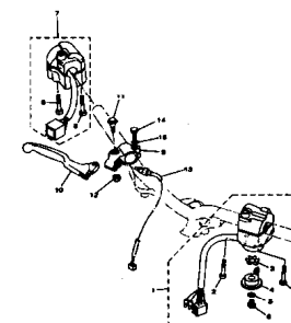
FIG.36 INTERRUPTOR DO GUIDÃO P.43
