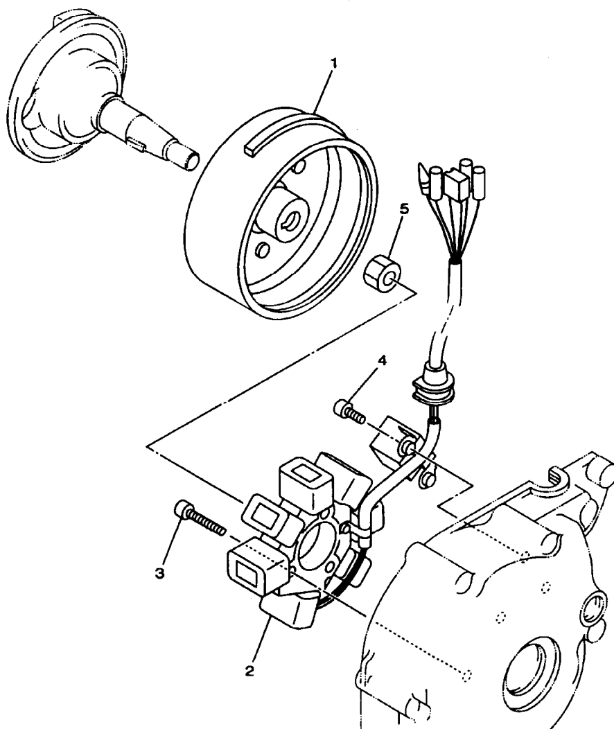
FIG. 30 - MAGNETO
