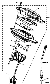
FIG.33 VELOCÍMETRO P.40
