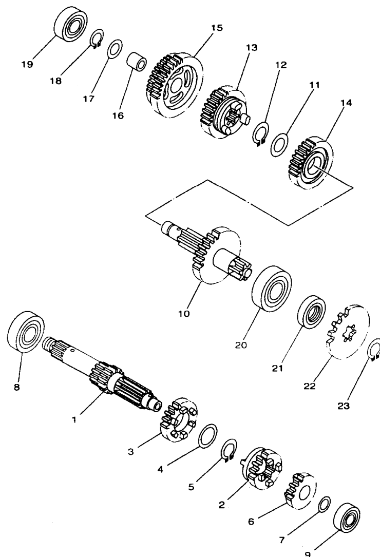
FIG. 14 - TRANSMISSÃO
