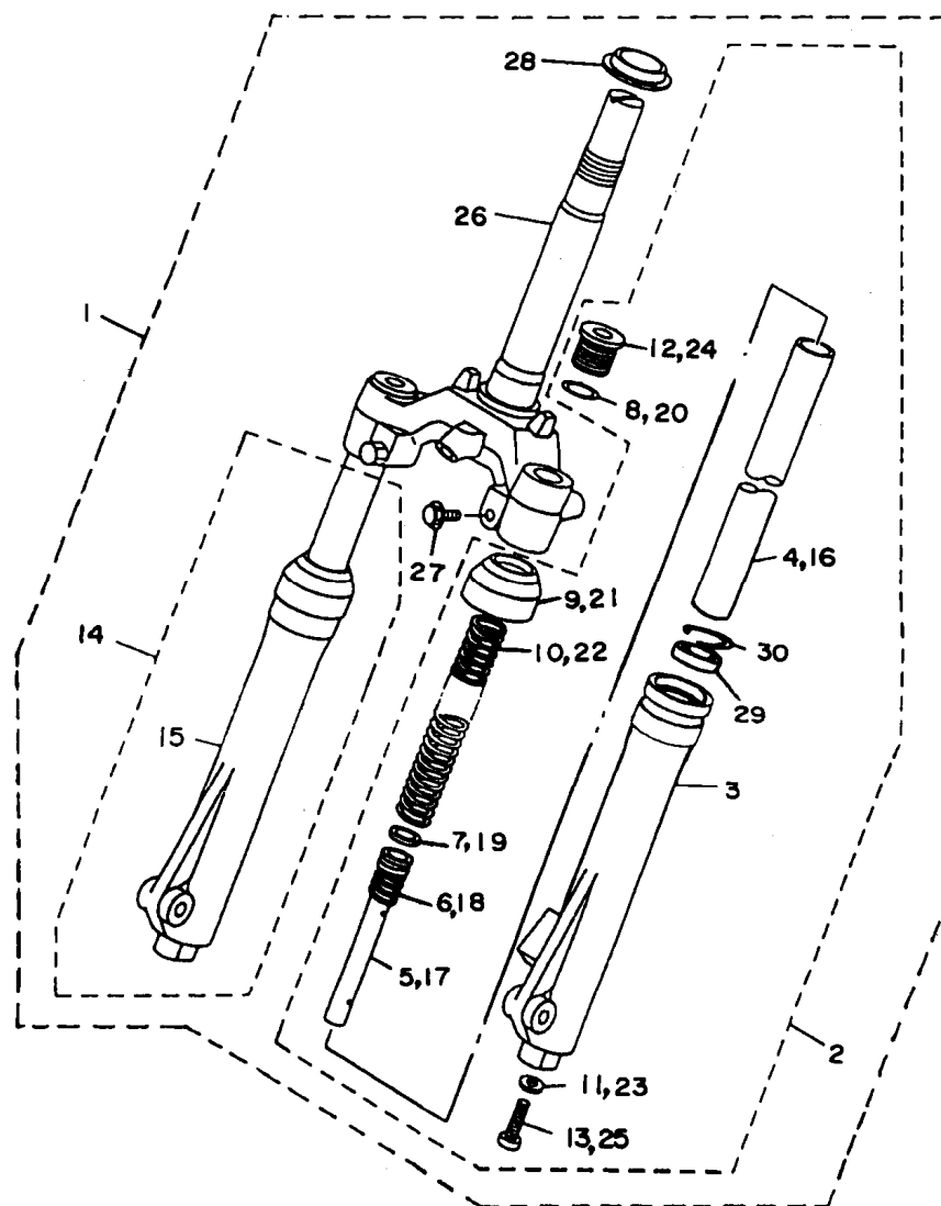
FIG. 22 - SUSPENSÃO DIANTEIRA
