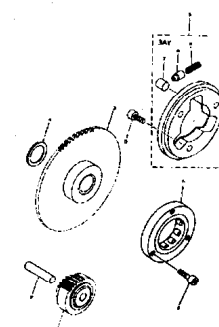
FIG.12 EMBREAGEM DA PARTIDA P.12
