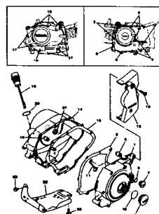
FIG.10 TAMPA DA CARCAÇA P.10
