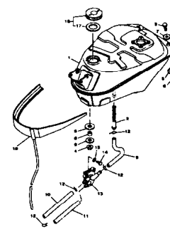
FIG.23 TANQUE DE COMBUSTÍVEL
