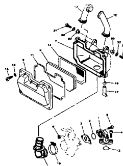
FIG.10 TAMPA DA CARCAÇA P.10
