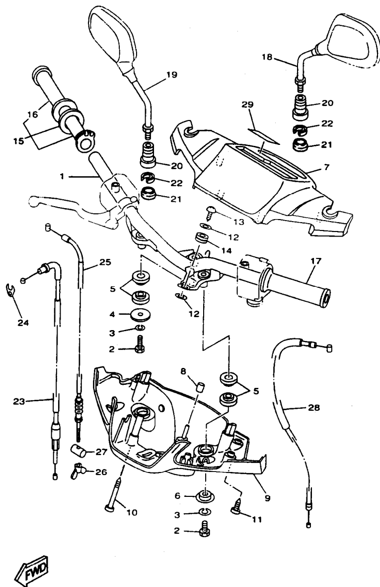
FIG. 27 - GUIDÃO E CABOS
