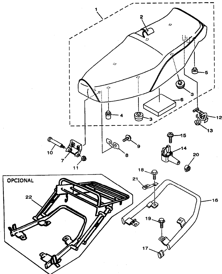
FIG. 24 - ASSENTO
