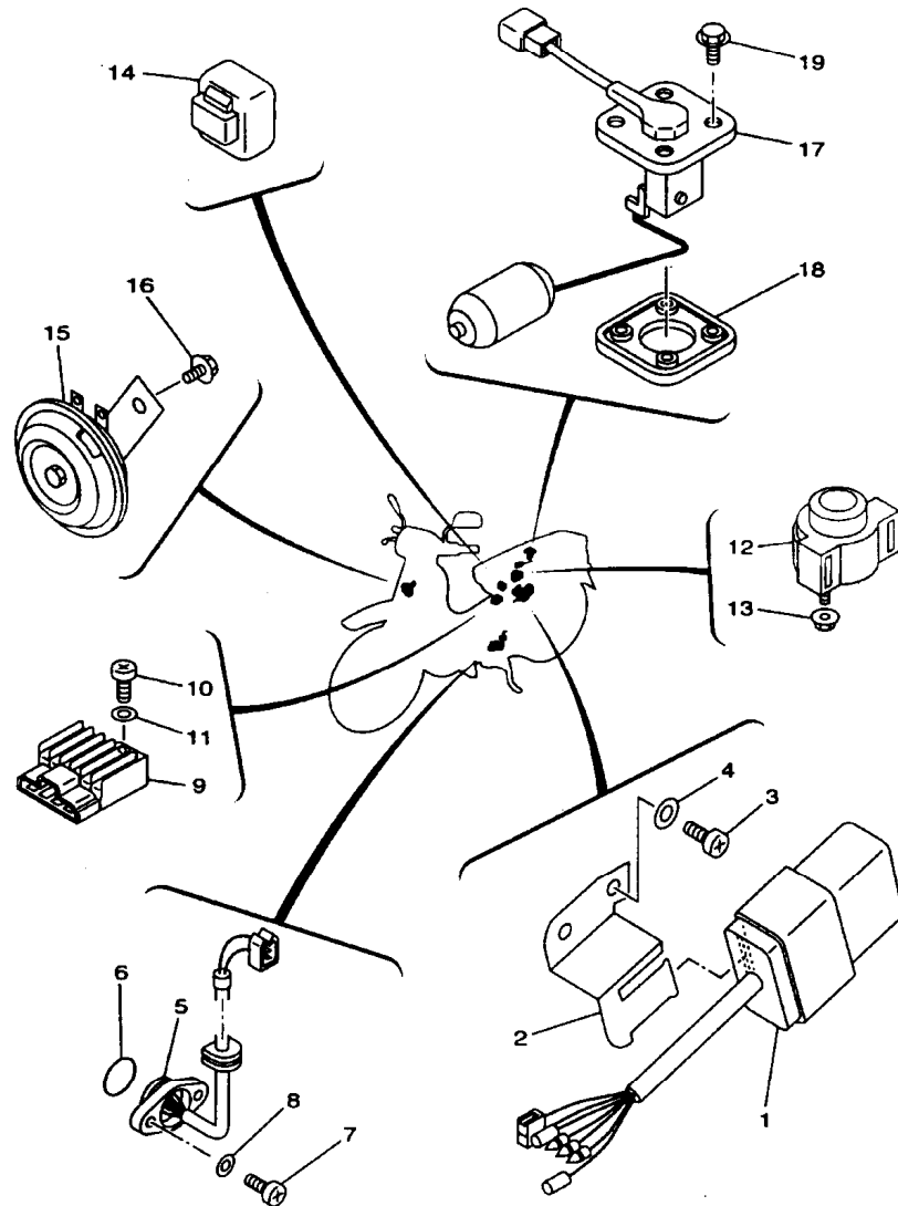
FIG. 38 - SISTEMA ELÉTRICO 2
