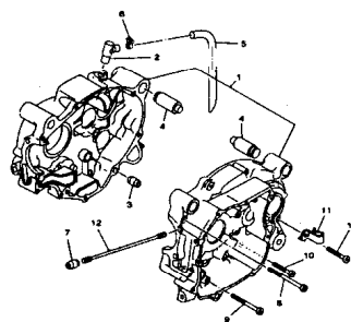
FIG.9 CARCAÇA DO MOTOR P.9
