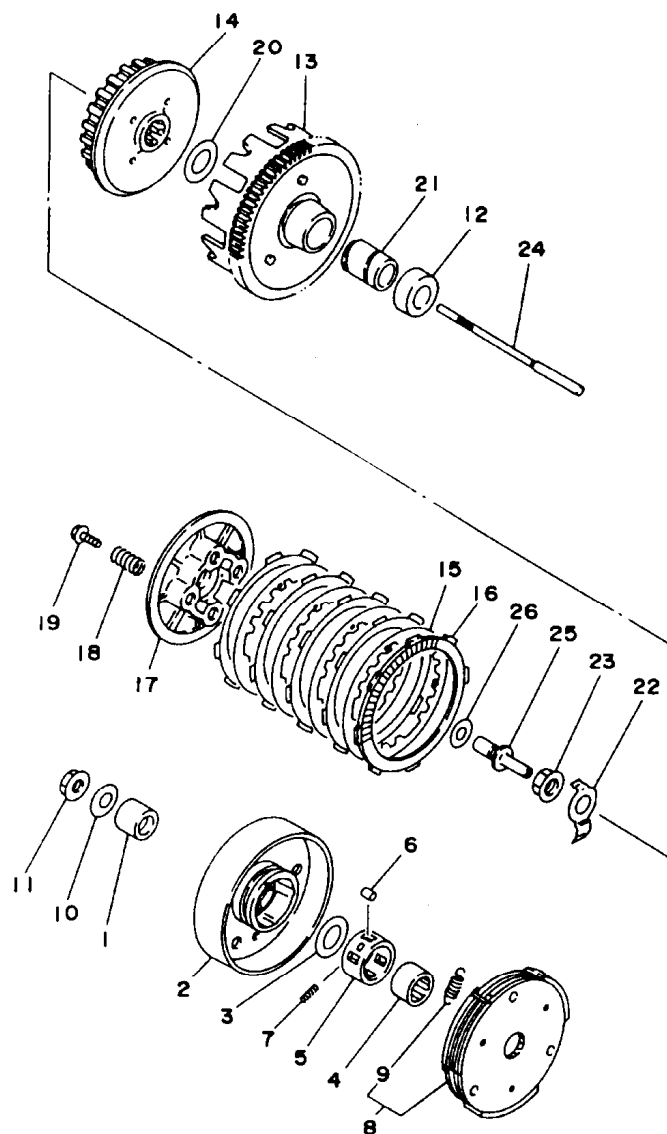
FIG. 13 - FRICÇÃO
