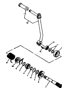
FIG.11 EIXO DE PARTIDA P.11
