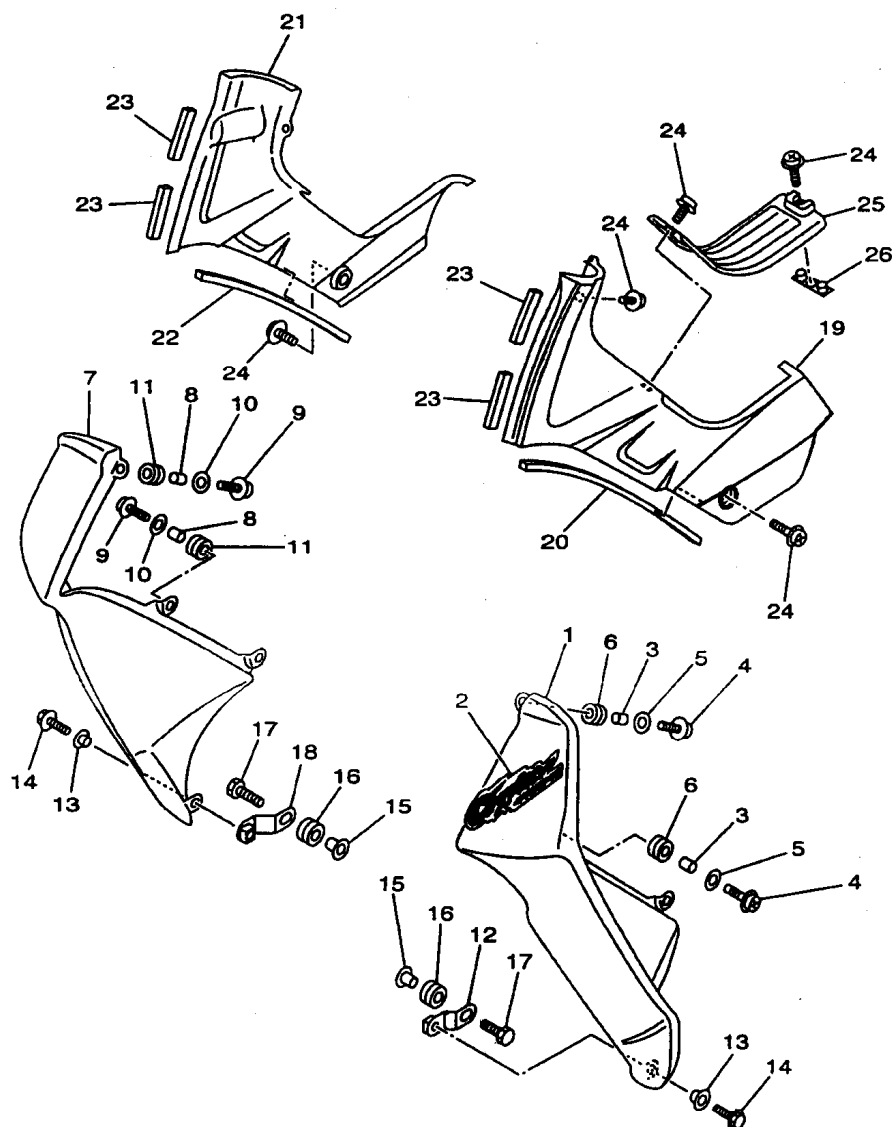
FIG. 29 - TAMPAS DIANTEIRAS
