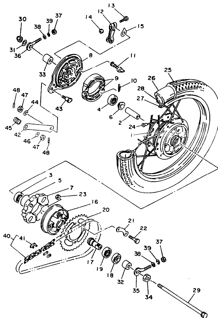
FIG. 26 - RODA TRASEIRA
