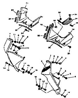
FIG.33 VELOCÍMETRO P.40
