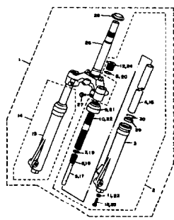
FIG.22 SUSPENSÃO DIANTEIRA
