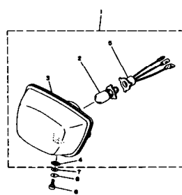
FIG.34 FAROL DIANTEIRO P.41
