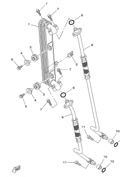
FIG. 7 COLETOR DE ÓLEO
