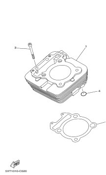
FIG. 2 CILINDRO
