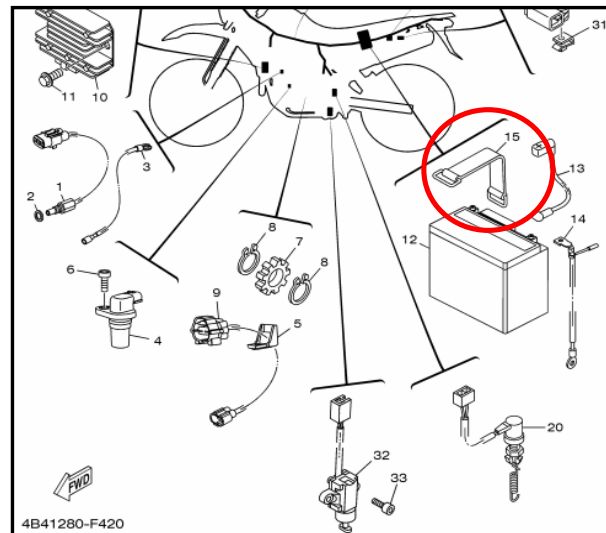
FIG. 42 SISTEMA ELÉTRICO 2
