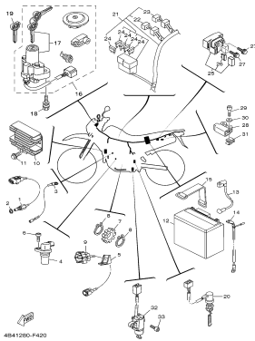
FIG. 42 SISTEMA ELÉTRICO 1
