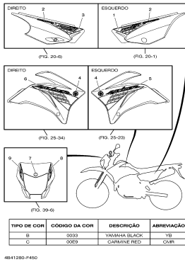
FIG. 45 GRÁFICOS. EMBLEMAS 2
