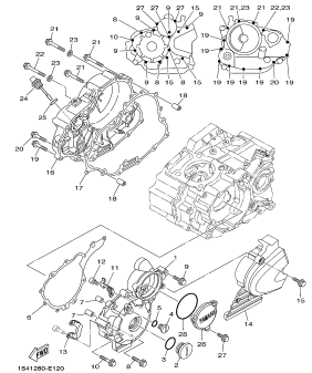
FIG. 12 TAMPA DA CARCAÇA
