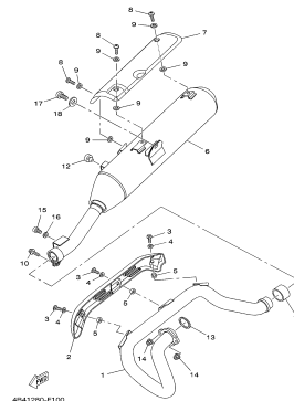
FIG. 10 ESCAPAMENTO
