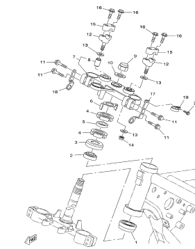
FIG. 23 MESA DO GUIDÃO P.29
