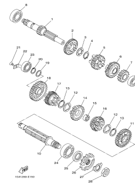
FIG. 15 TRANSMISSÃO P.20
