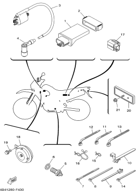
FIG. 43 SISTEMA ELÉTRICO 2
