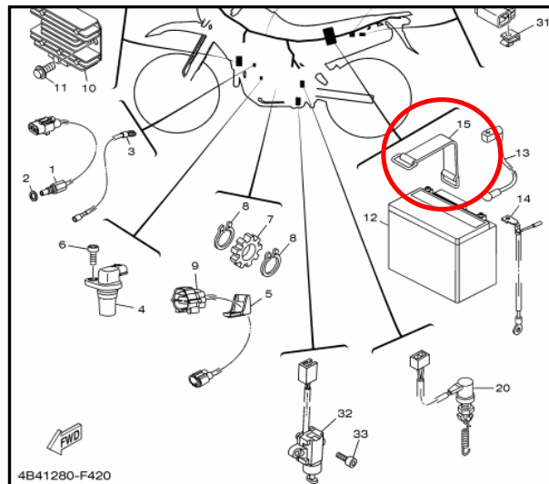
FIG. 42 SISTEMA ELÉTRICO 2
