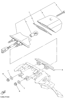
FIG. 40 LANTERNA TRASEIRA
