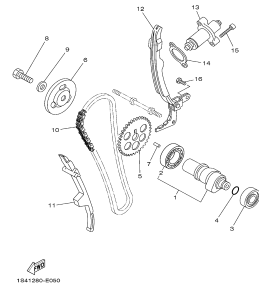
FIG. 9 ADMISSÃO 2
