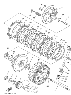
FIG. 14 EMBREAGEM P.18
