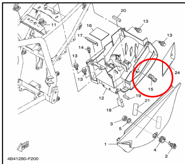
FIG. 20 TAMPAS LATERAIS
