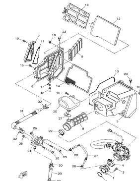
FIG. 8 ADMISSÃO
