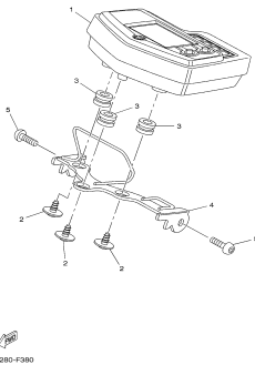
FIG. 42 SISTEMA ELÉTRICO 1
