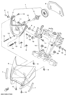
FIG. 39 FAROL DIANTEIRO
