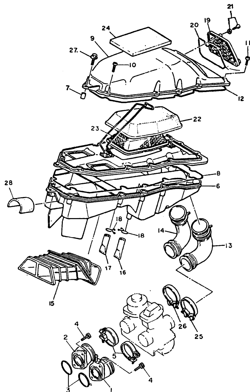
FIG. 07 - ENTRADA DE AR
