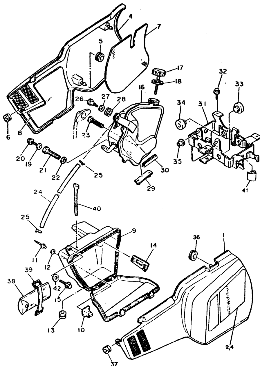
FIG. 19 - TAMPA LATERAL
