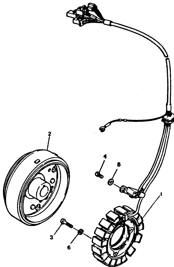
FIG. 32 - MAGNETO
