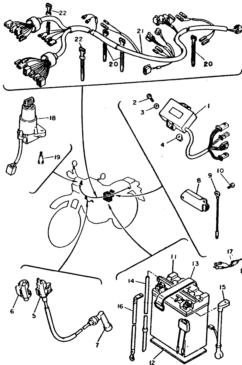
FIG. 38 - ELÉTRICA 1
