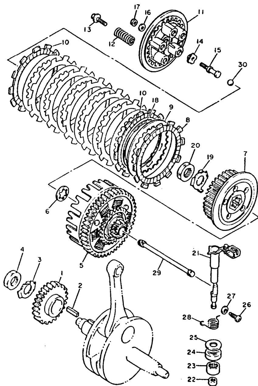
FIG. 13 - FRICÇÃO
