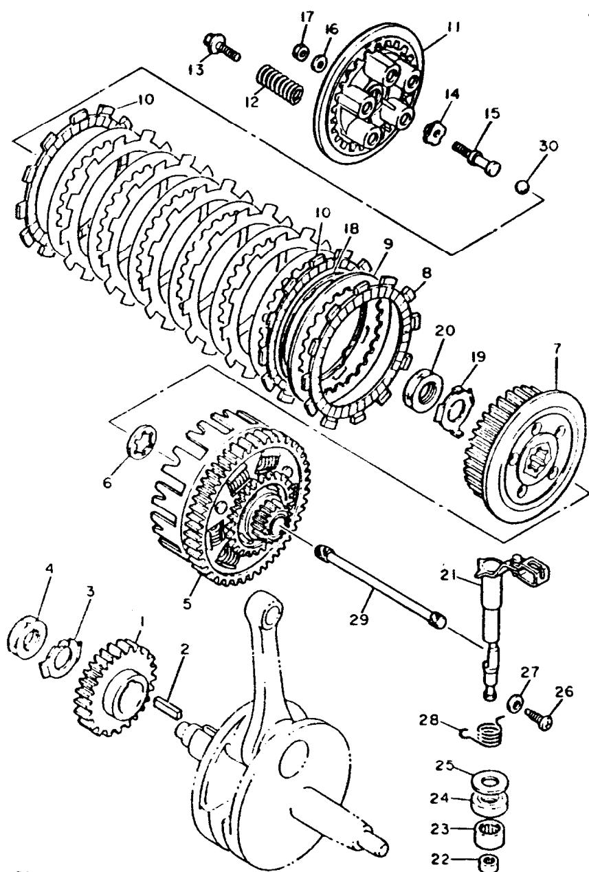
FIG. 13 - FRICÇÃO
