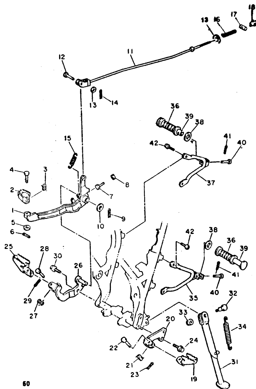
FIG. 30 - PEDAL DE FREIO, ESTRIBO E CAVALETE LATERAL
