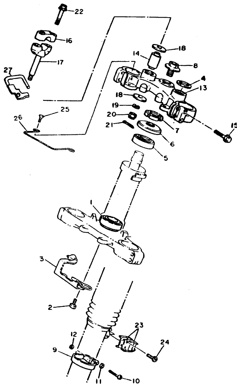
FIG. 22 - DIREÇÃO
