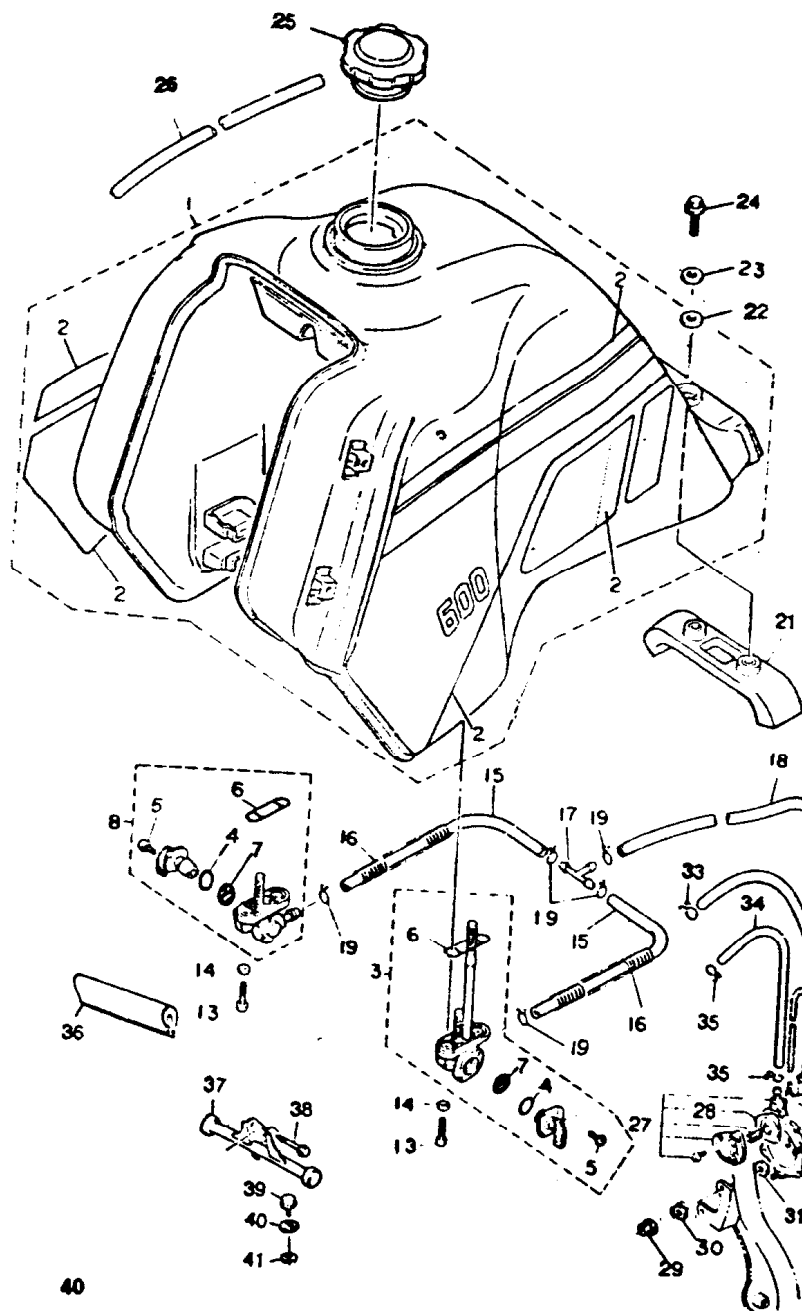
FIG. 24 - TANQUE DE GASOLINA
