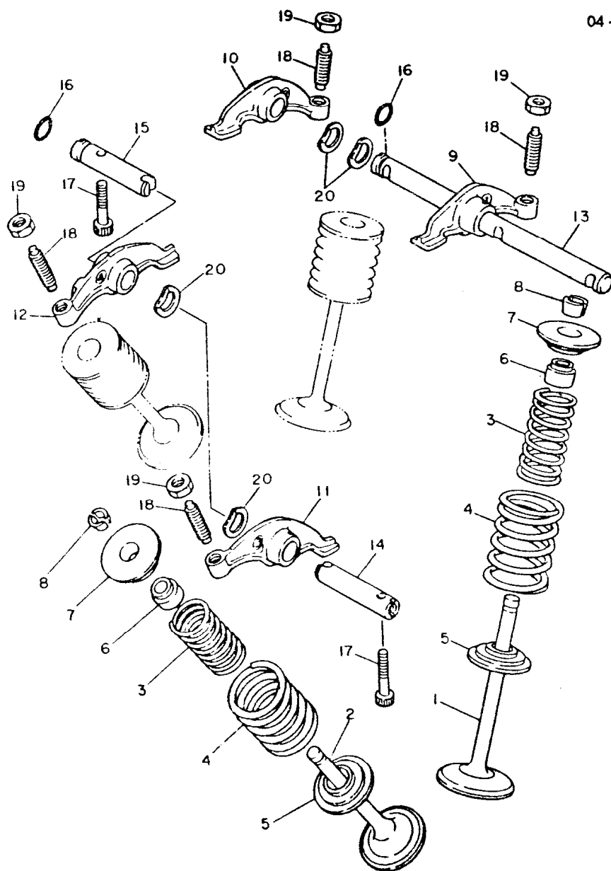
FIG. 04 - VÁLVULA
