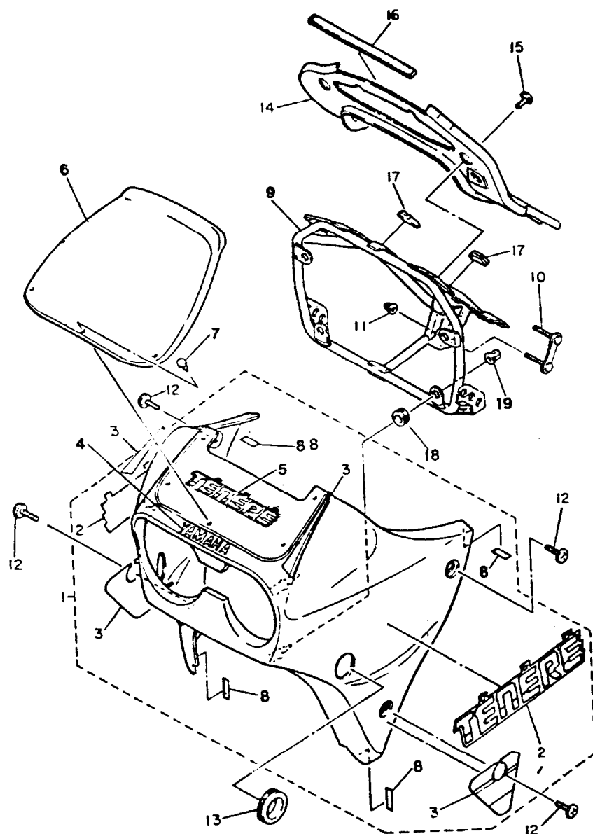
FIG. 31 - CARENAGEM
