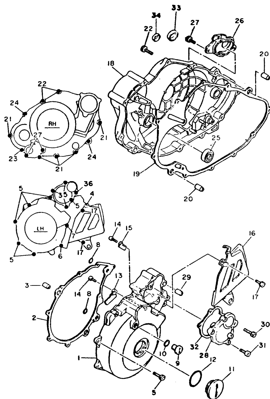
FIG. 11 - TAMPA DA CARÇAÇA
