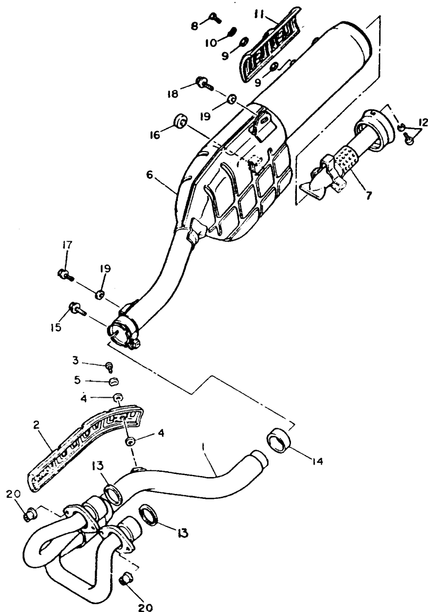
FIG. 09 - ESCAPAMENTO
