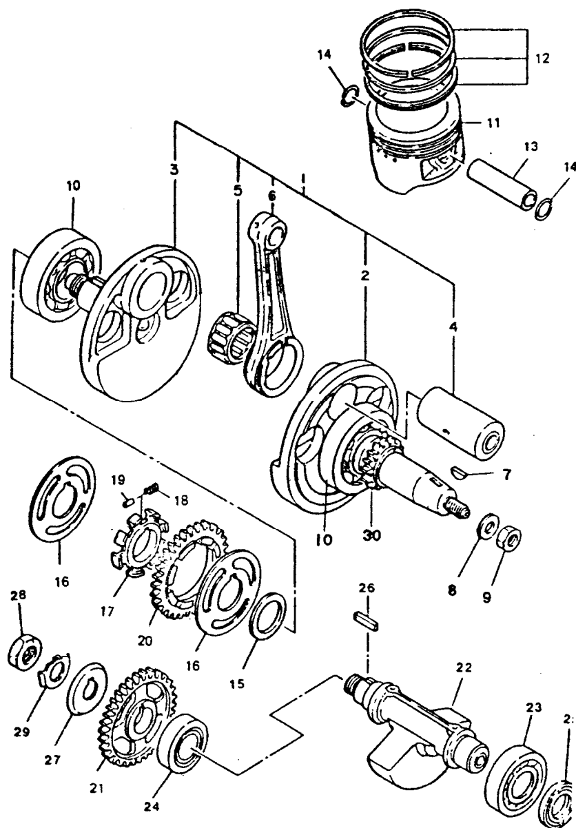
FIG. 03 - VIRABREQUIM E PISTÃO
