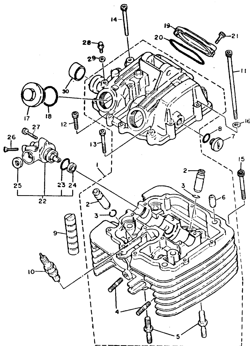
FIG. 1 - CABEÇOTE DO CILINDRO
