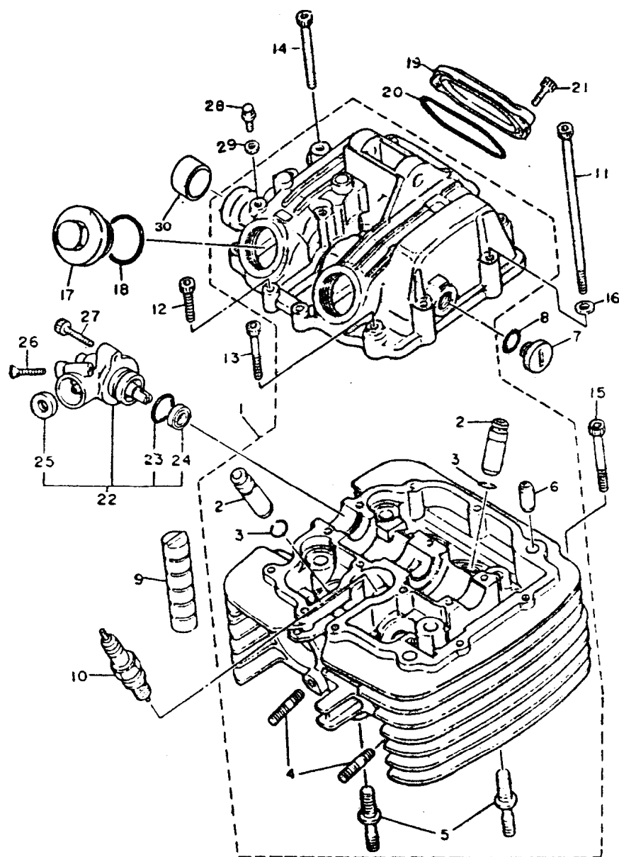
FIG. 01 - CABEÇOTE DO CILINDRO
