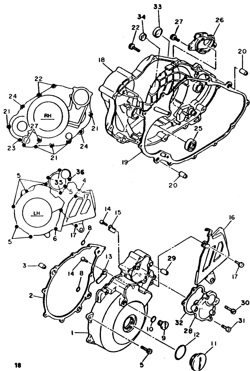
FIG. 11 - TAMPA DA CARCAÇA
