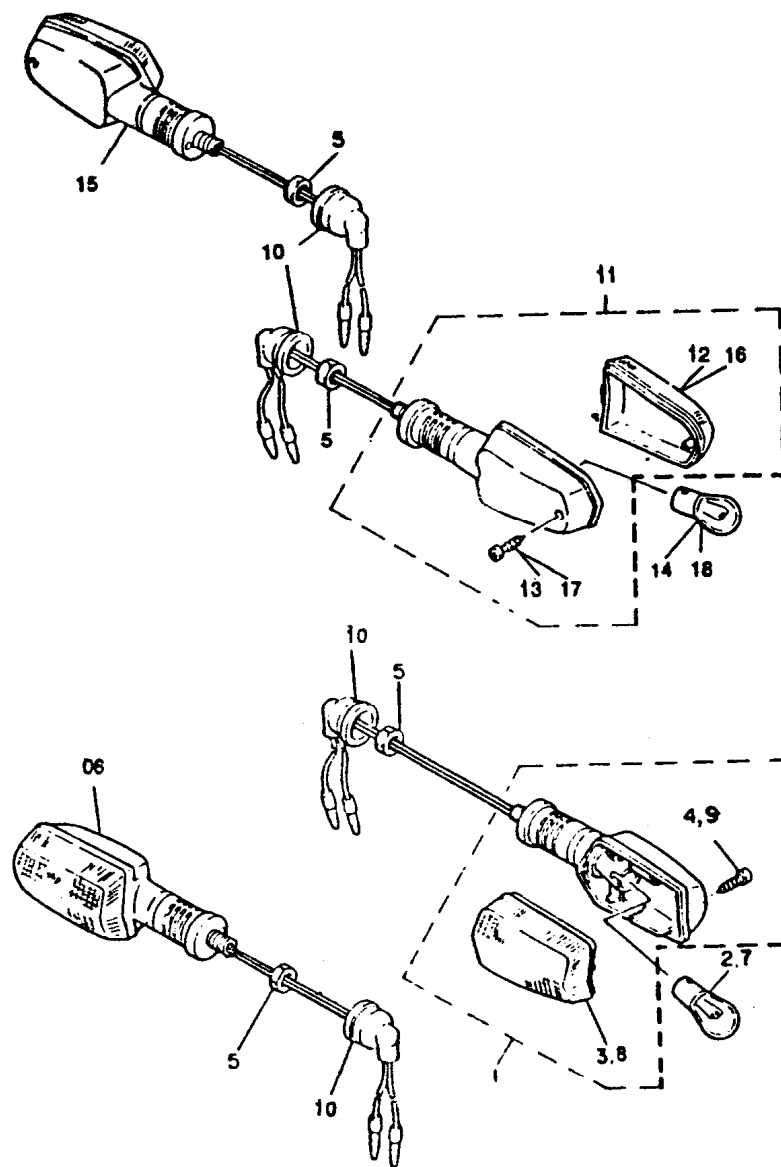
FIG. 33 - PISCA-PISCA
