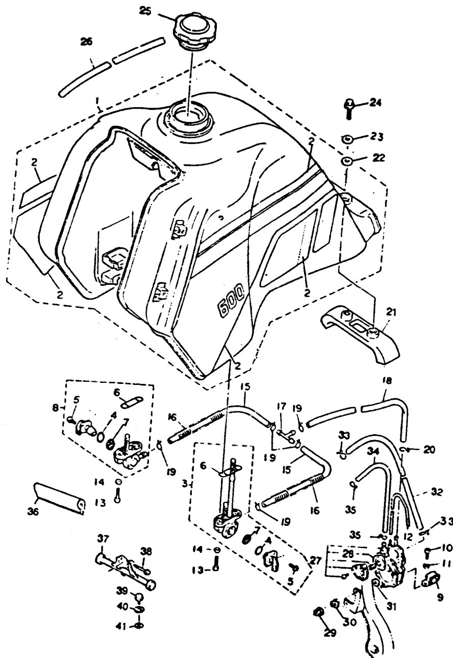
FIG. 24 - TANQUE DE GASOLINA
