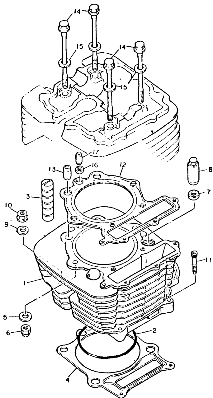
FIG. 02 - CILINDRO DO MOTOR
