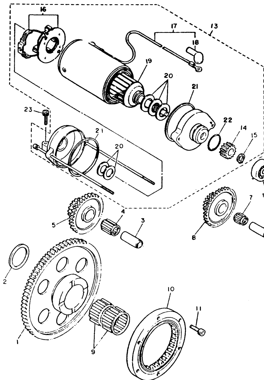
FIG. 12 - MOTOR DE PARTIDA
