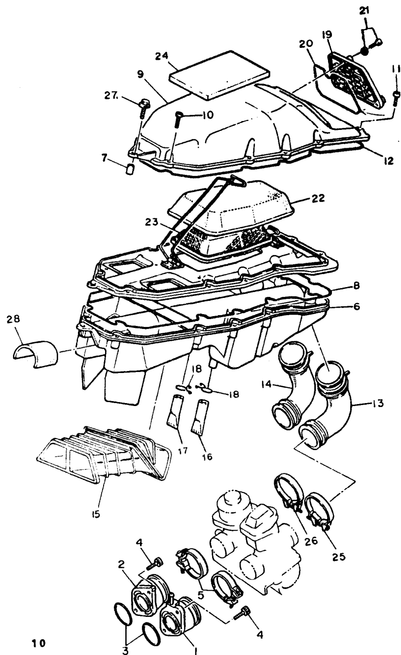
FIG. 07 - ENTRADA DE AR
