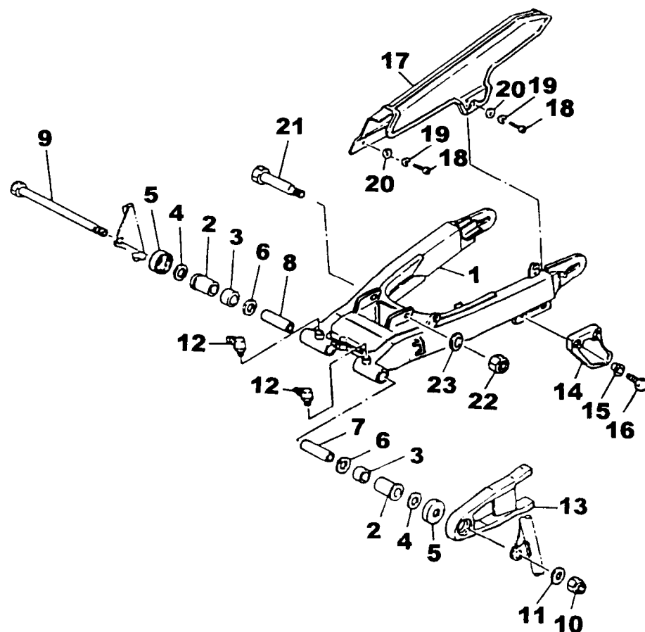
FIG. 19 - GARFO TRASEIRO
