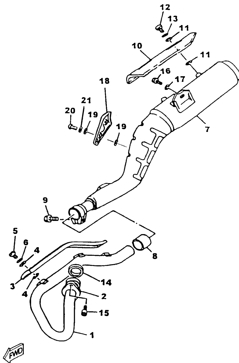
FIG. 08 - ESCAPAMENTO
