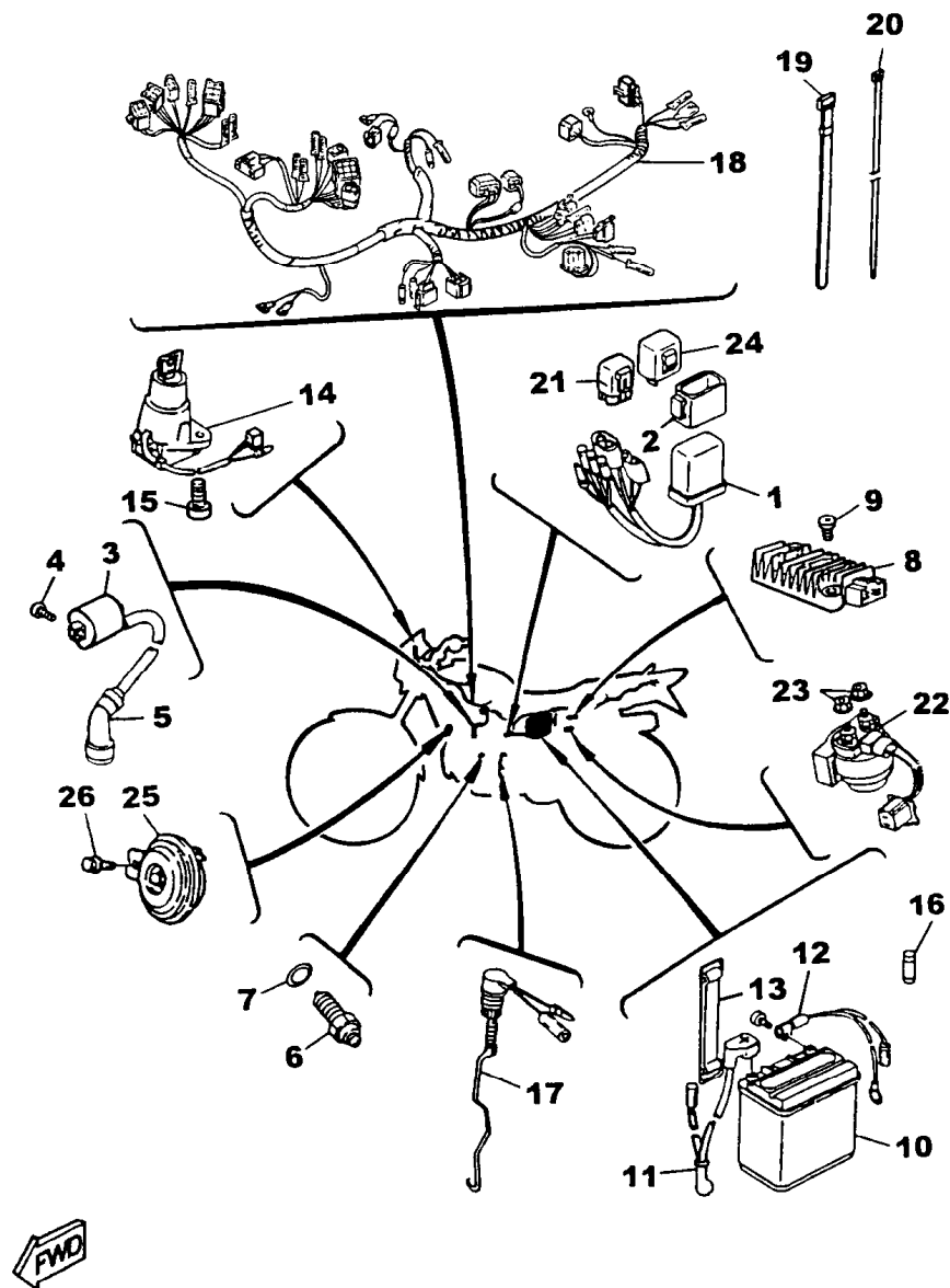
FIG. 41 - SISTEMA ELÉTRICO
