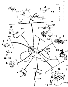
FIG.41 SISTEMA ELÉTRICO
