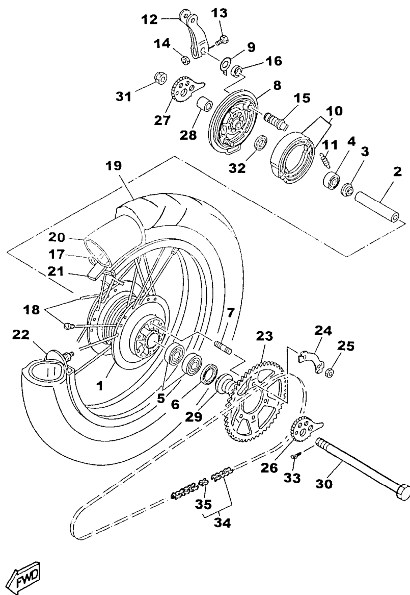
FIG. 24 - RODA TRASEIRA
