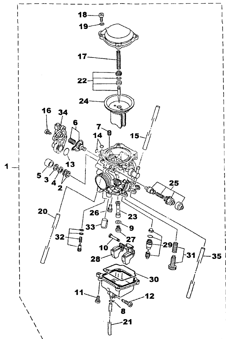
FIG. 16 - CARBURADOR
