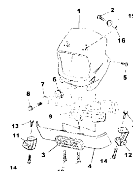
FIG.28 CARENAGEM P.30
