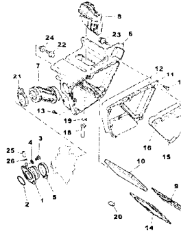
FIG.7 FILTRO DE AR P.8
