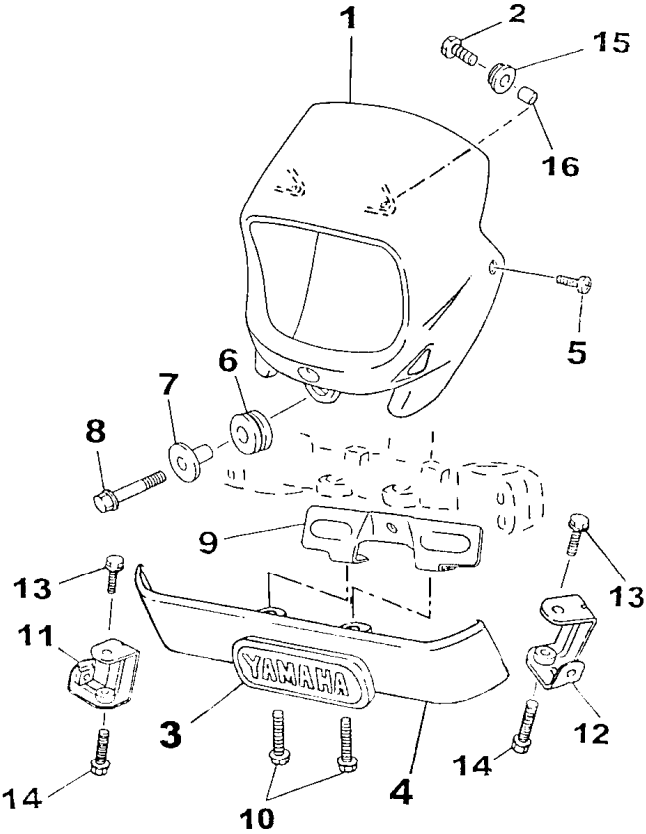
FIG. 28 - CARENAGEM
