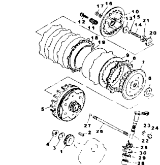
FIG.12 FRICÇÃO P.13
