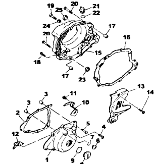
FIG.10 TAMPA DA CARCAÇA P.11
