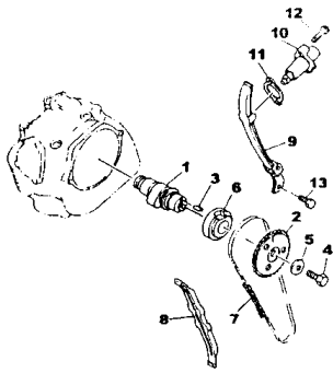
FIG.5 EIXO DE COMANDO P.6
