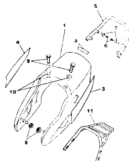
FIG.30 TAMPATRASEIRA • SUPORTE DO CARONA P.32
