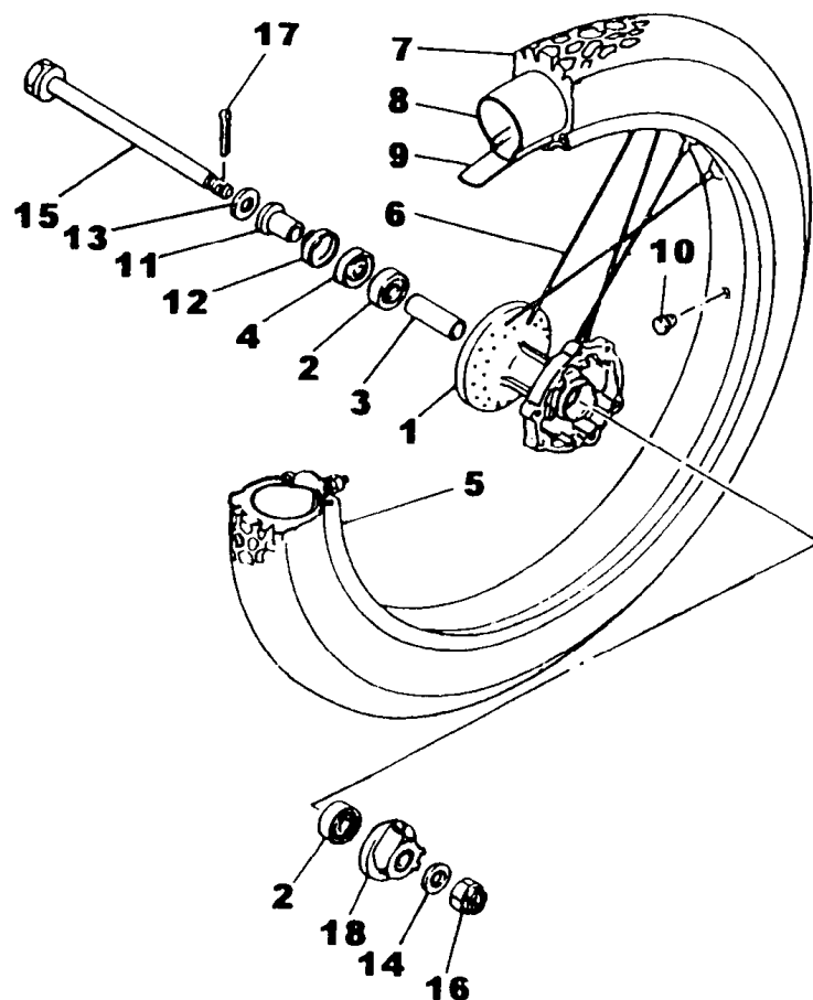
FIG. 22 - RODA DIANTEIRA
