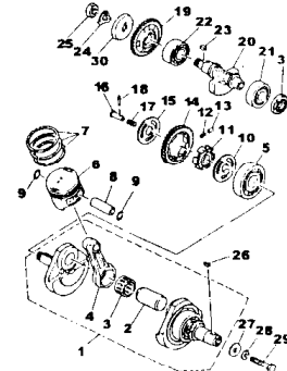
FIG.3 VIRABREQUIM E PISTÃO P.3
