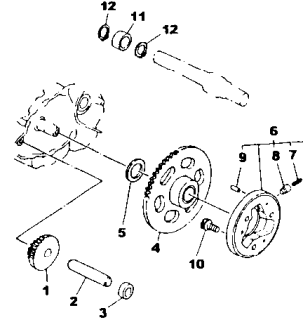
FIG.11 EMBREAGEM DE PARTIDA P.12
