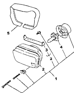
FIG.34 FAROL DIANTEIRO P.37
