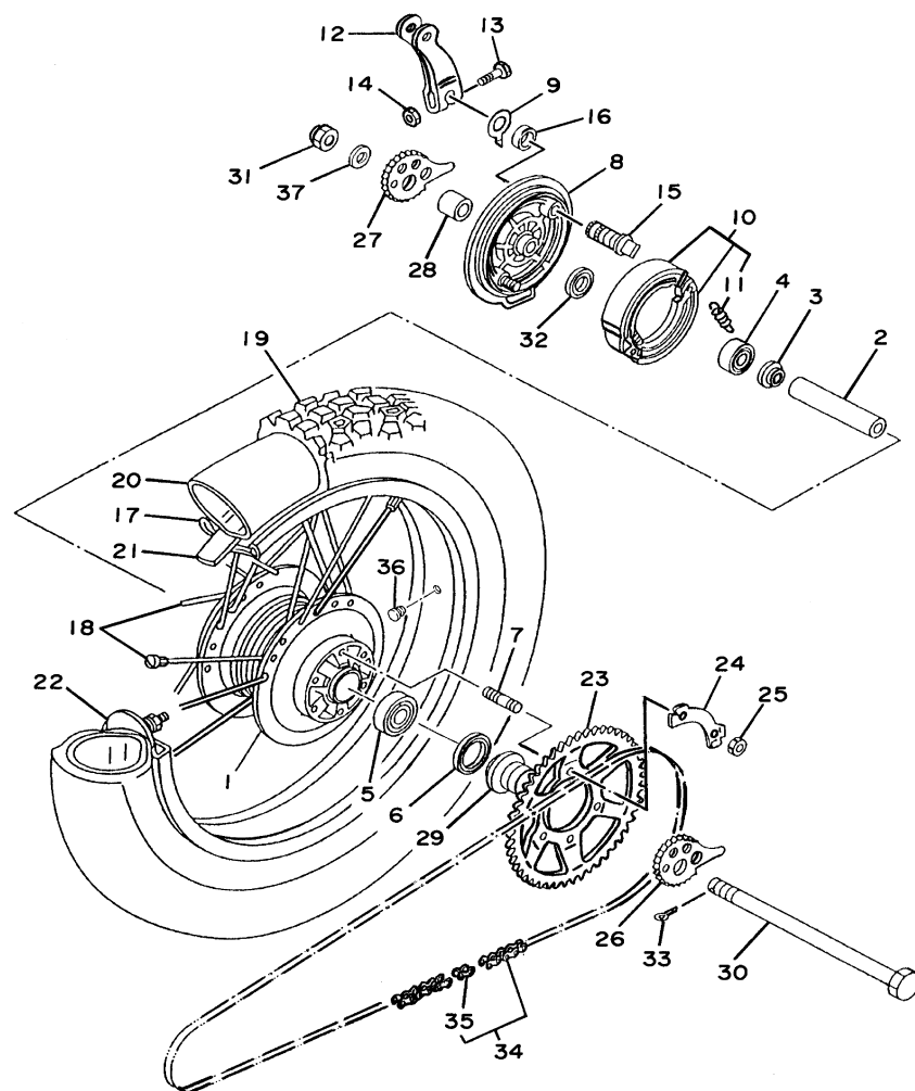
FIG. 28 RODA TRASEIRA
