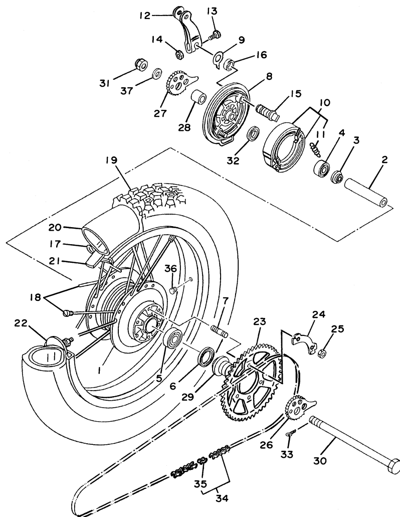
FIG. 28 - RODA TRASEIRA
