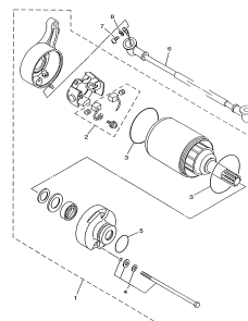
FIG.34 MOTOR DE PARTIDA
