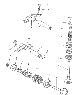
FIG.4 VÁLVULAS P.06
