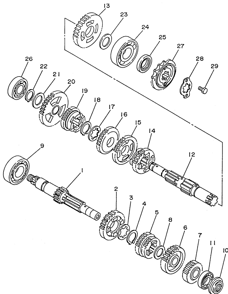
FIG. 14 - TRANSMISSÃO
