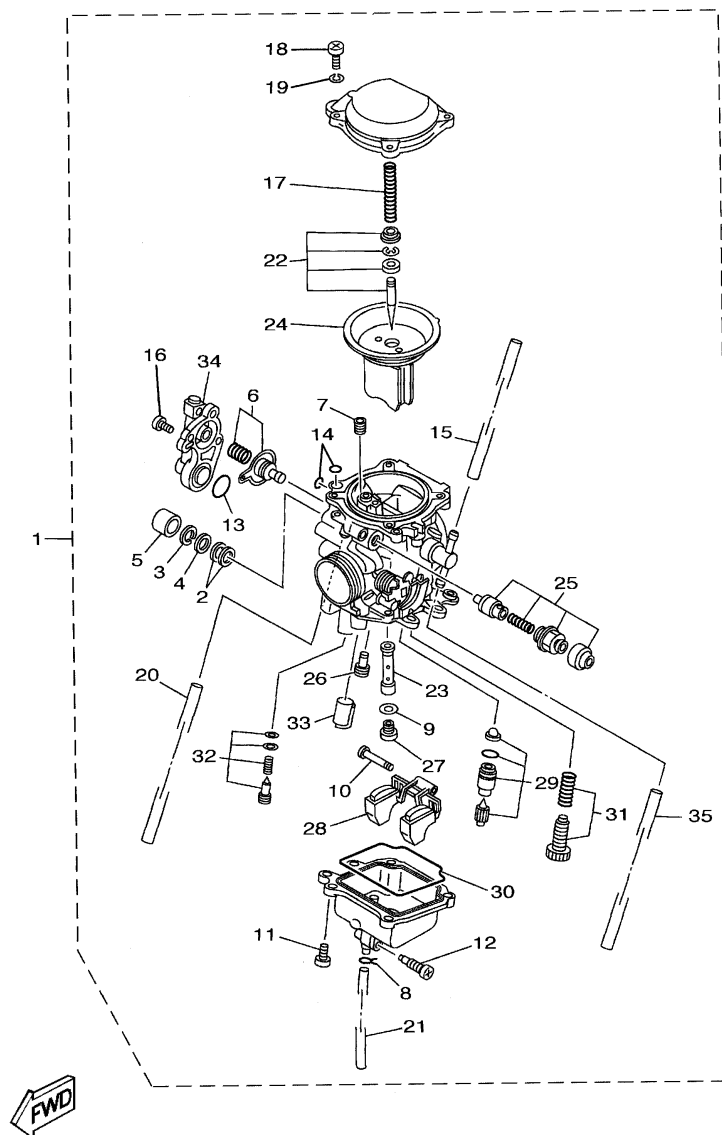
FIG. 08 - CARBURADOR
