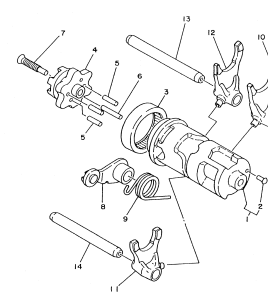
FIG.15 EIXO TRAMBULADOR P.21
