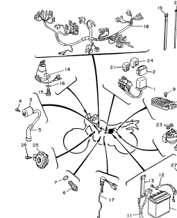
FIG.40 SISTEMA ELÉTRICO P.50
