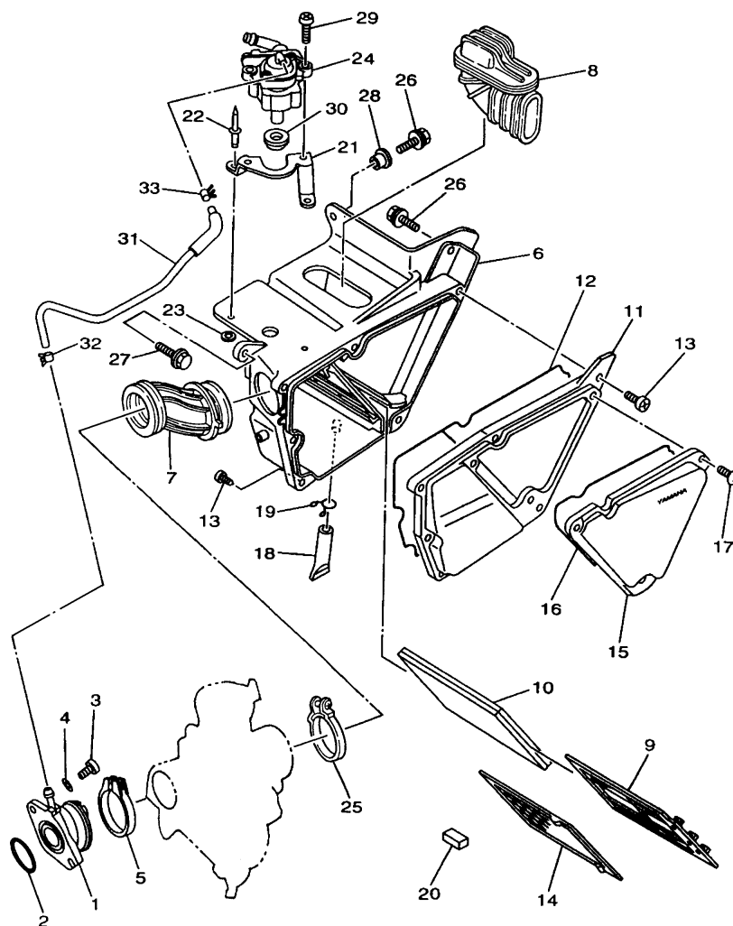
FIG. 07 - FILTRO DE AR
