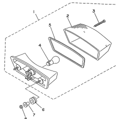
FIG.38 LANTERNA TRASEIRA P.48
