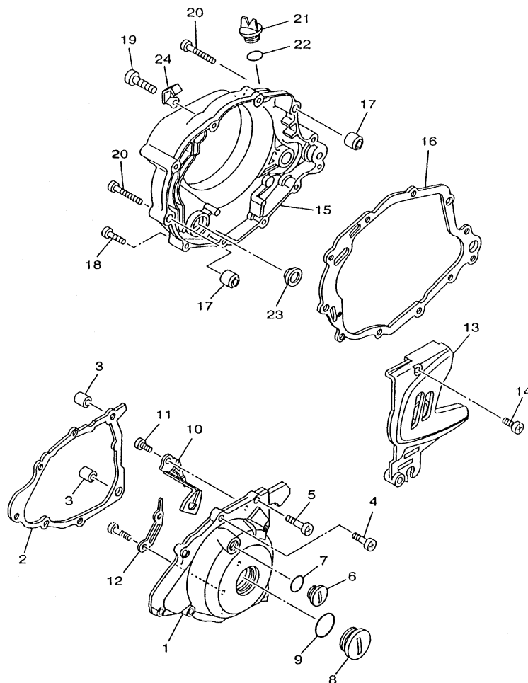
FIG. 11 - TAMPA DA CARÇAÇA
