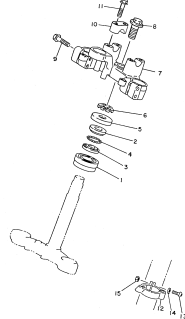
FIG.22 MESA DO GUIDÃO P.29
