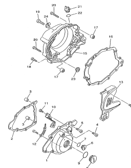
FIG.11 TAMPA DA CARCAÇA P.15
