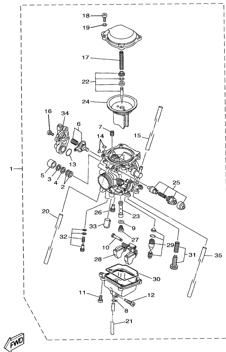
FIG. 08 - CARBURADOR
