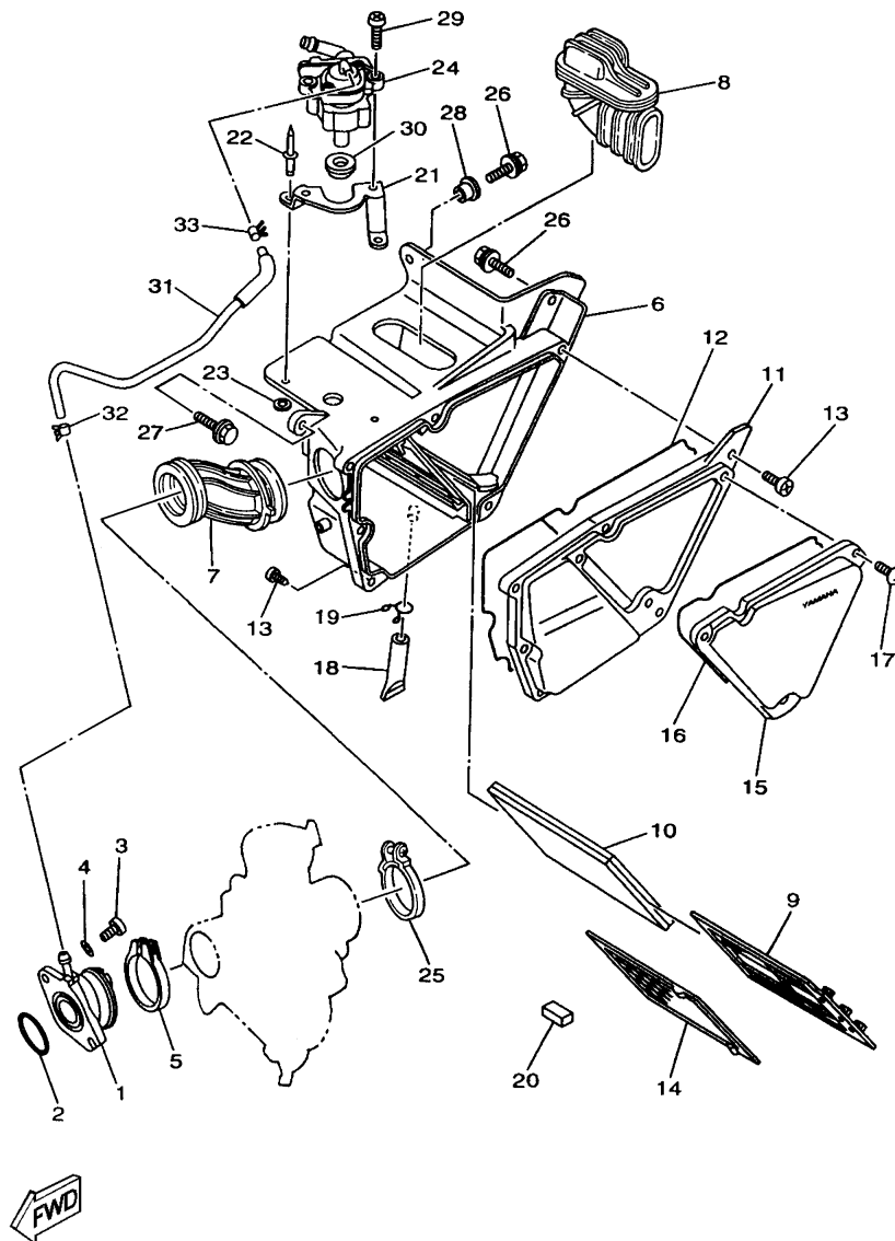
FIG. 07 - FILTRO DE AR
