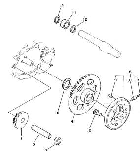
FIG.12 EMBREAGEM DE PARTIDA P.16
