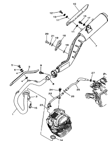
FIG.9 ESCAPAMENTO P.13
