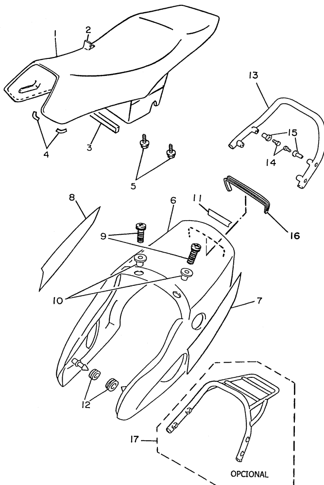
FIG. 25 - ASSENTO
