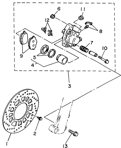
FIG. 27 - DISCO E PINÇA DO FREIO
