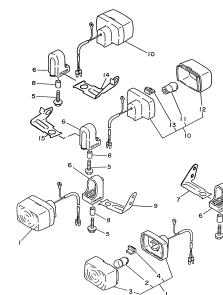
FIG.35 SINALIZADORES (PISCA-PISCA)
