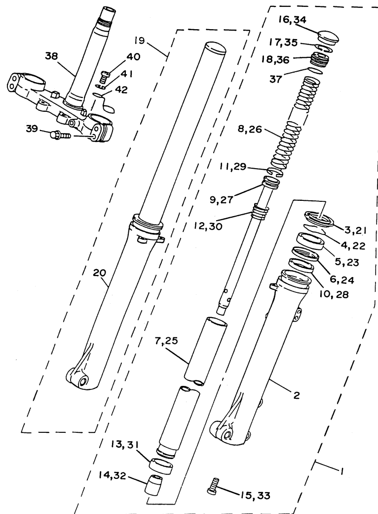
FIG. 23 - GARFO DIANTEIRO
