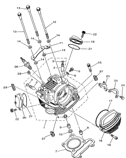
FIG.1 CABEÇOTE DO CILINDRO e P.02
