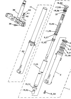
FIG.23 GARFO DIANTEIRO P.30 e P.31
