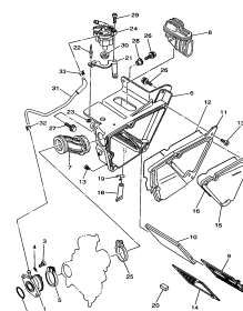
FIG.7 FILTRO DE AR P.09 e P.10
