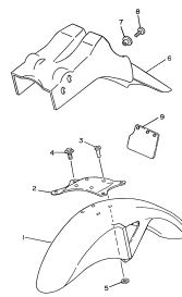
FIG.18 PÁRA-LAMAS DIANTEIRO E TRASEIRO P.25
