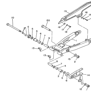
FIG.20 GARFO TRASEIRO P. 27
