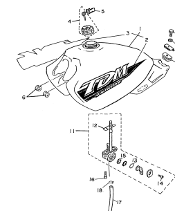
FIG.24 TANQUE DE COMBUSTÍVEL P.32
