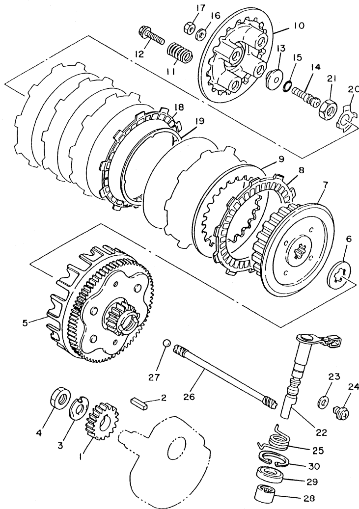
FIG. 13 - FRICÇÃO
