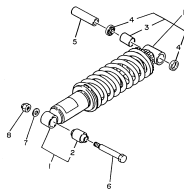
FIG.21 AMORTECEDOR TRASEIRO P.28
