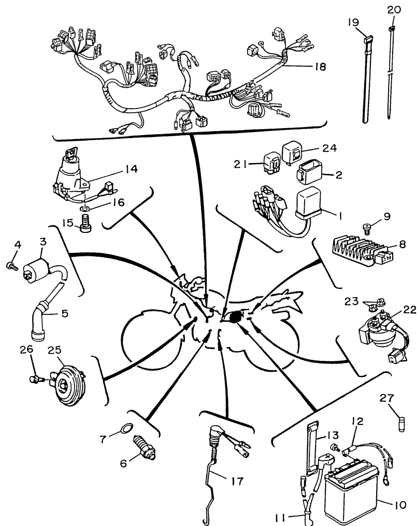
FIG. 40 - SISTEMA ELÉTRICO
