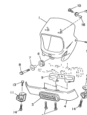
FIG.32 CARENAGEM
