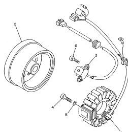
FIG.33 CONJUNTO MAGNETO
