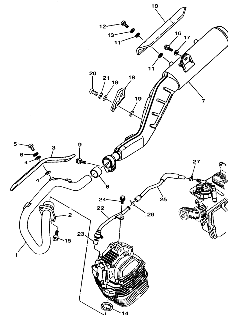
FIG. 09 - ESCAPAMENTO
