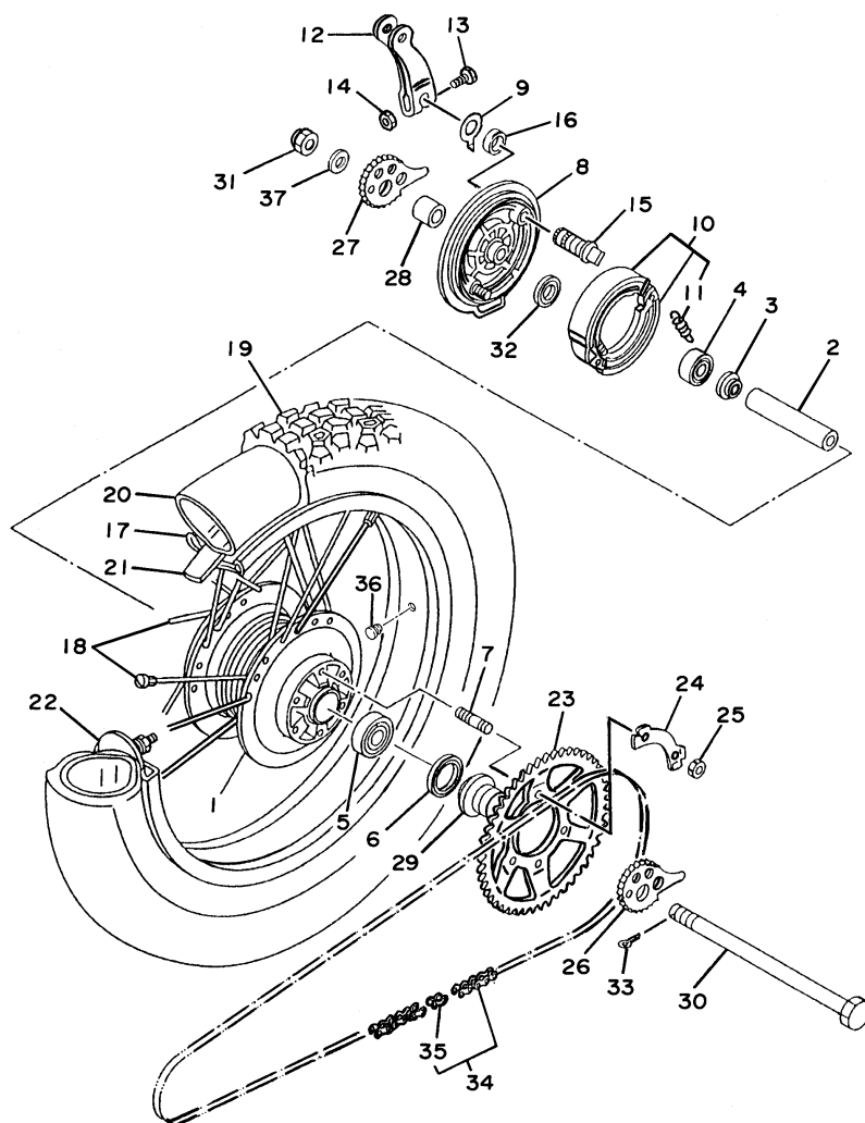
FIG. 28 - RODA TRASEIRA
