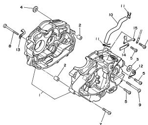
FIG.10 CARCAÇA DO MOTOR P.14
