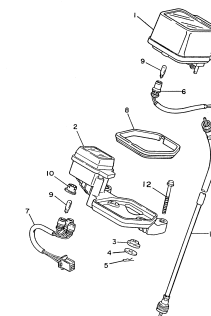
FIG.36 VELOCÍMETRO
