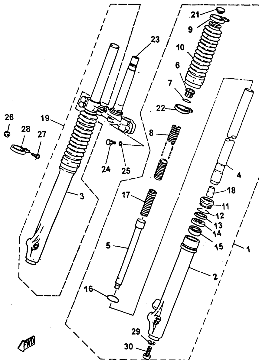
FIG. 22 - GARFO TELESCÓPICO
