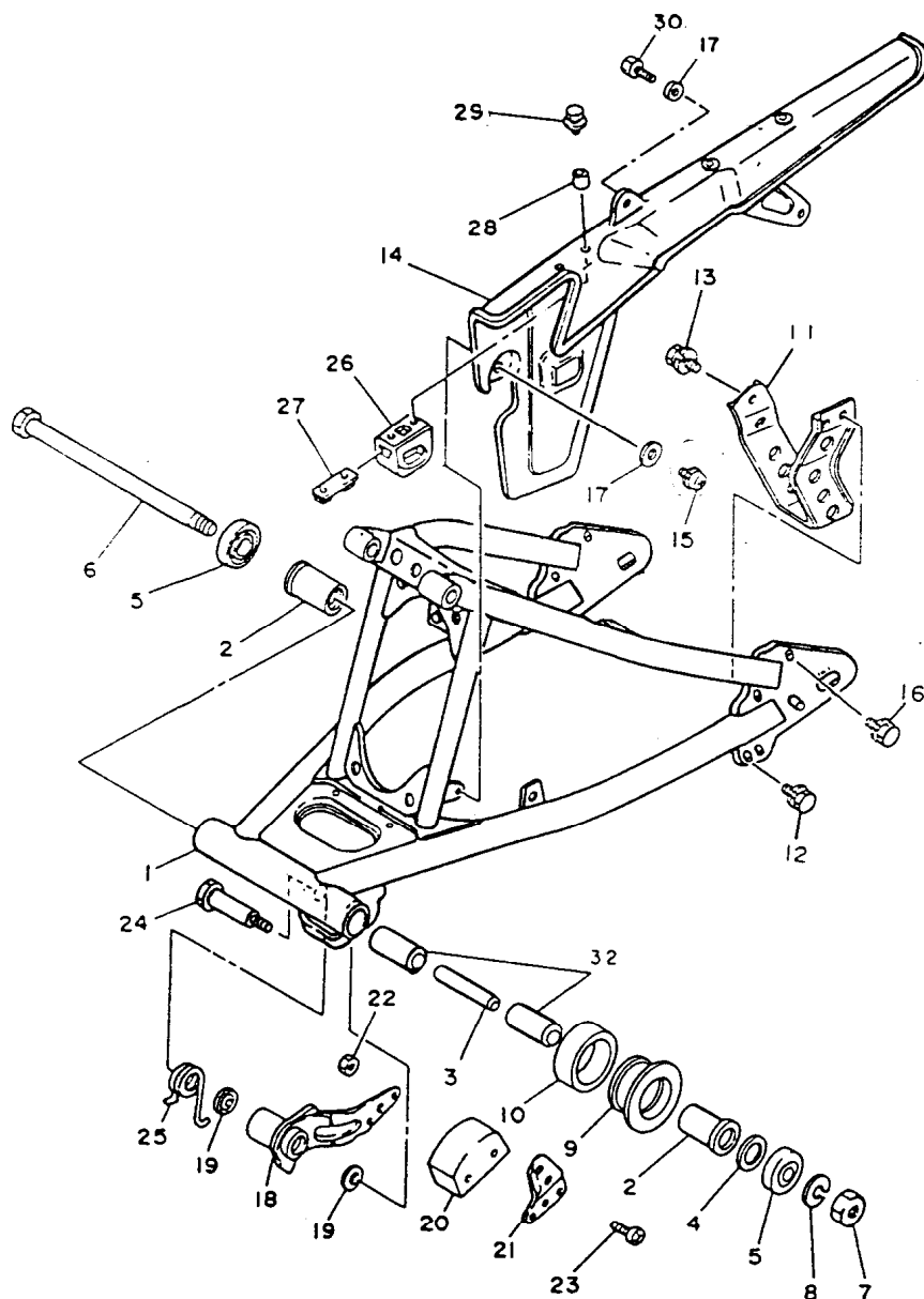
FIG. 18 - GARFO TRASEIRO
