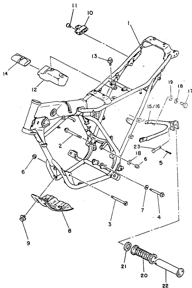
FIG. 17 - CHASSI
