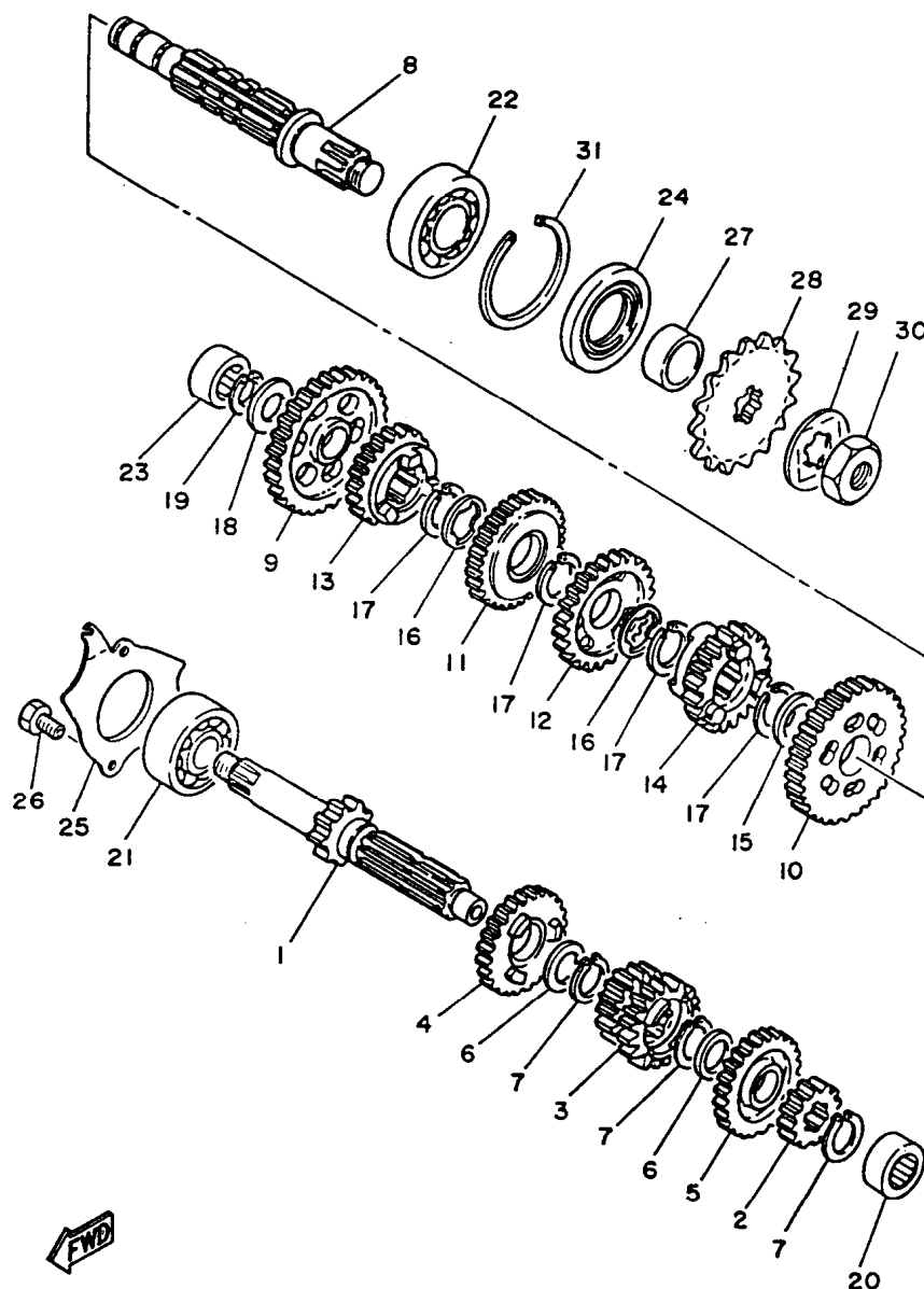
FIG. 06 - TRANSMISSÃO
