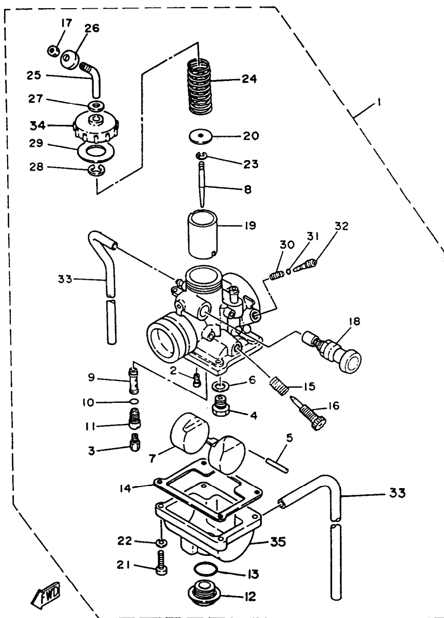
FIG. 12 - CARBURADOR
