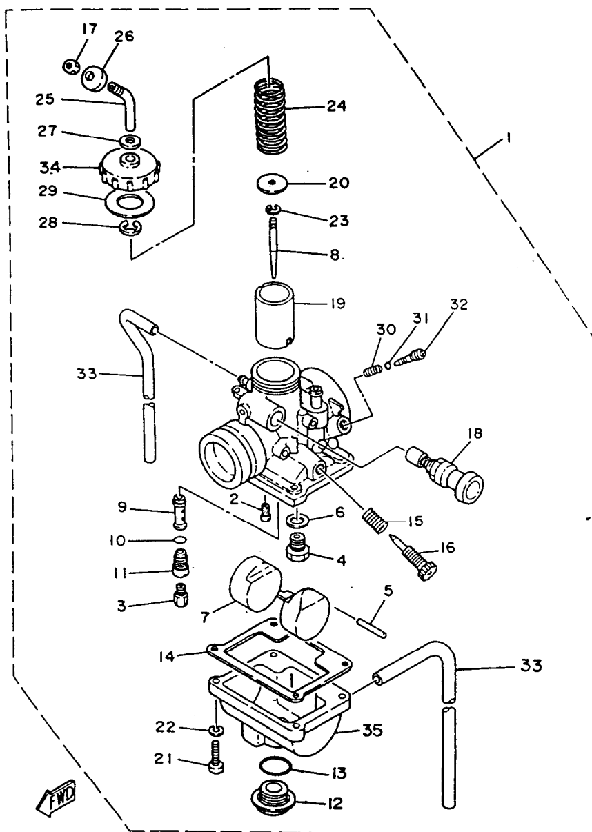
FIG. 12 - CARBURADOR
