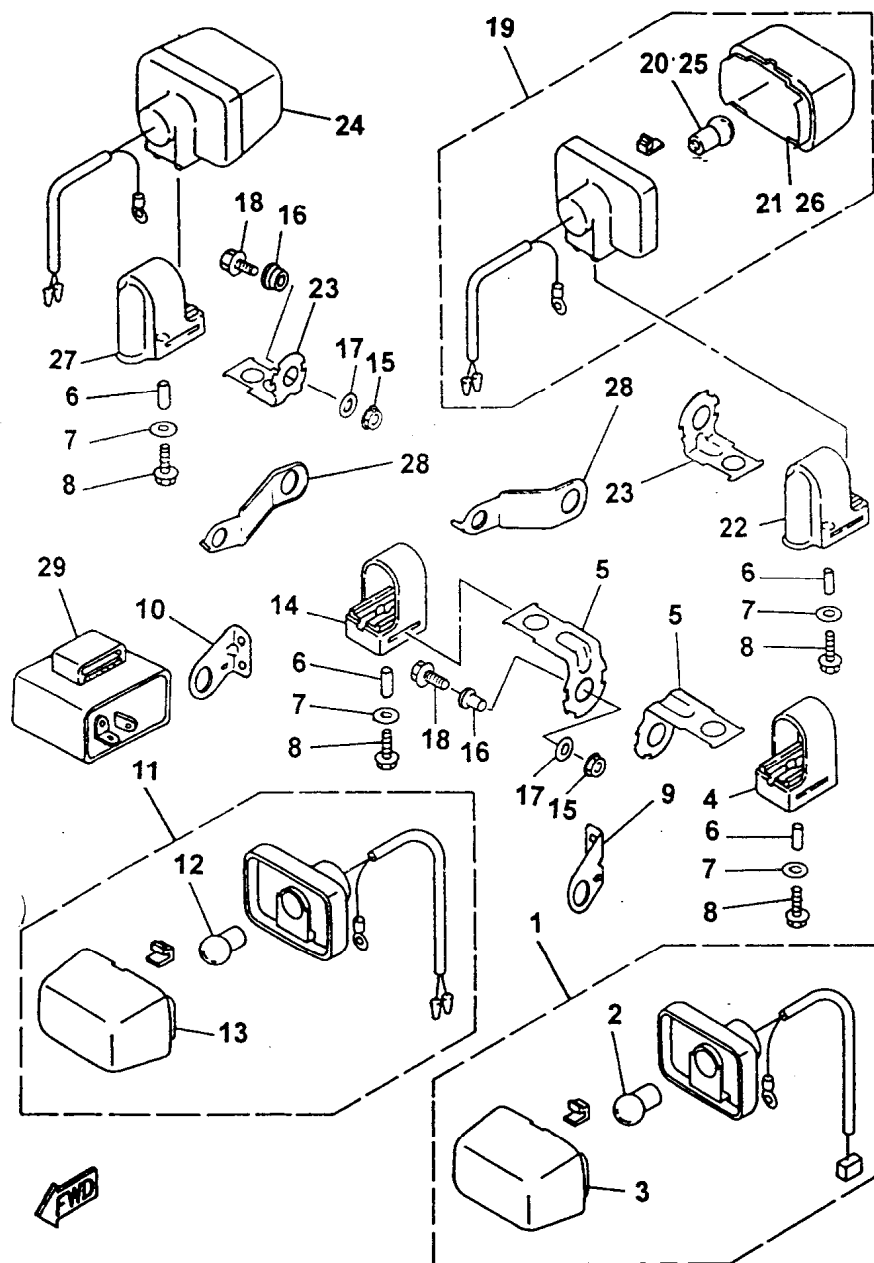
FIG. 31 - SINALIZADORES (PISCA-PISCA)
