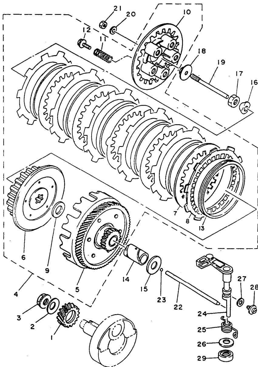
FIG. 05 - FRICÇÃO
