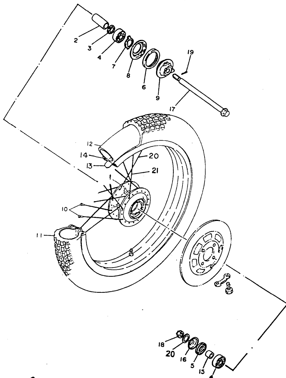
FIG. 28 - RODA DIANTEIRA
