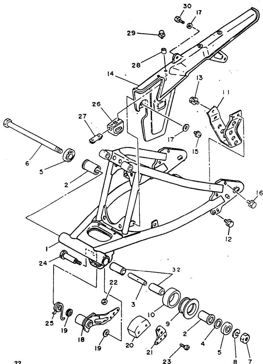
FIG. 18 - GARFO TRASEIRO
