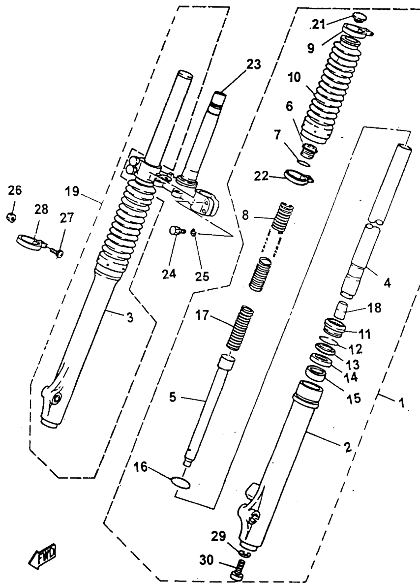
FIG. 22 - GARFO TELESCÓPICO
