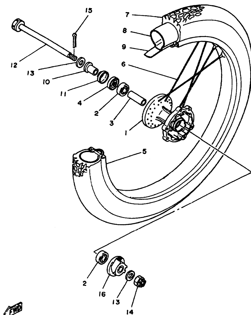
FIG. 27 - RODA DIANTEIRA
