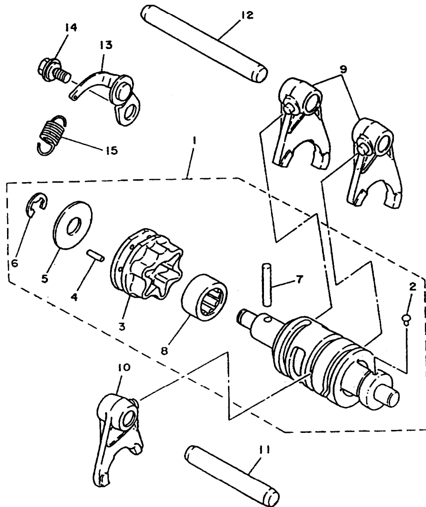
FIG. 07 - EIXO TRAMBULADOR
