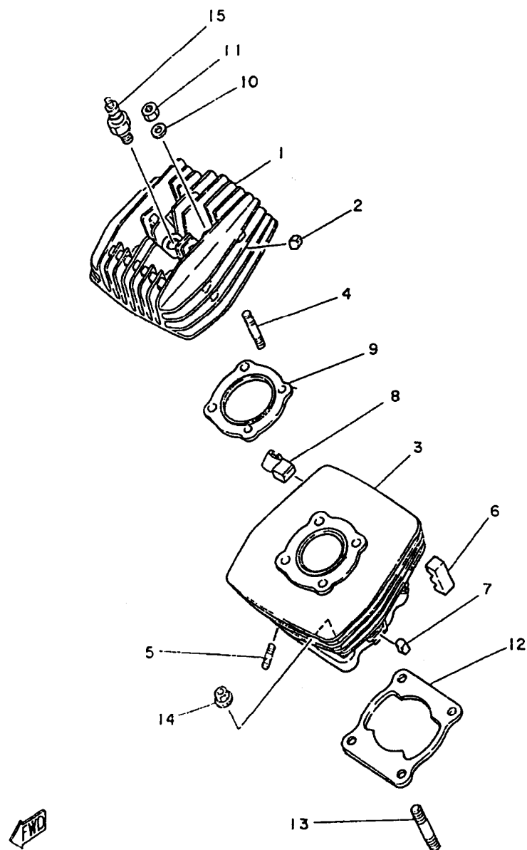
FIG. 01 - CABEÇOTE E CILINDRO
