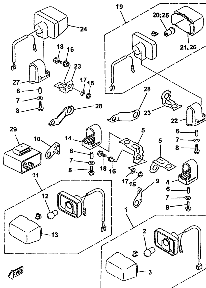
FIG. 30 - SINALIZADORES (PISCA-PISCA)
