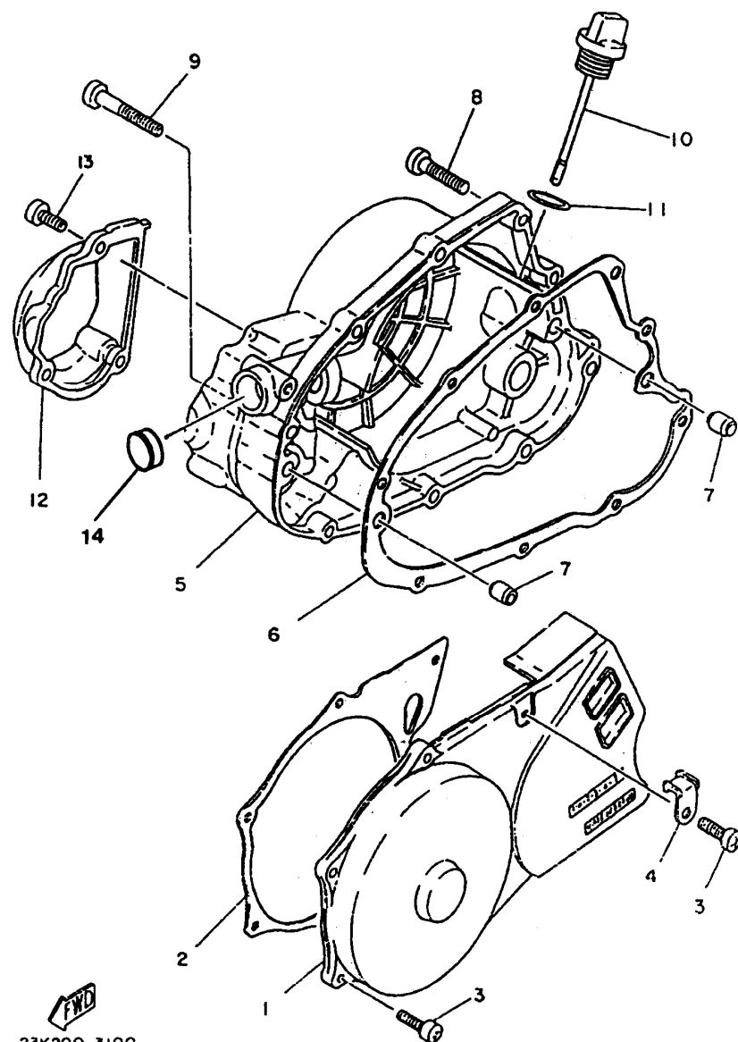
FIG. 03 - TAMPA DA CARCAÇA
