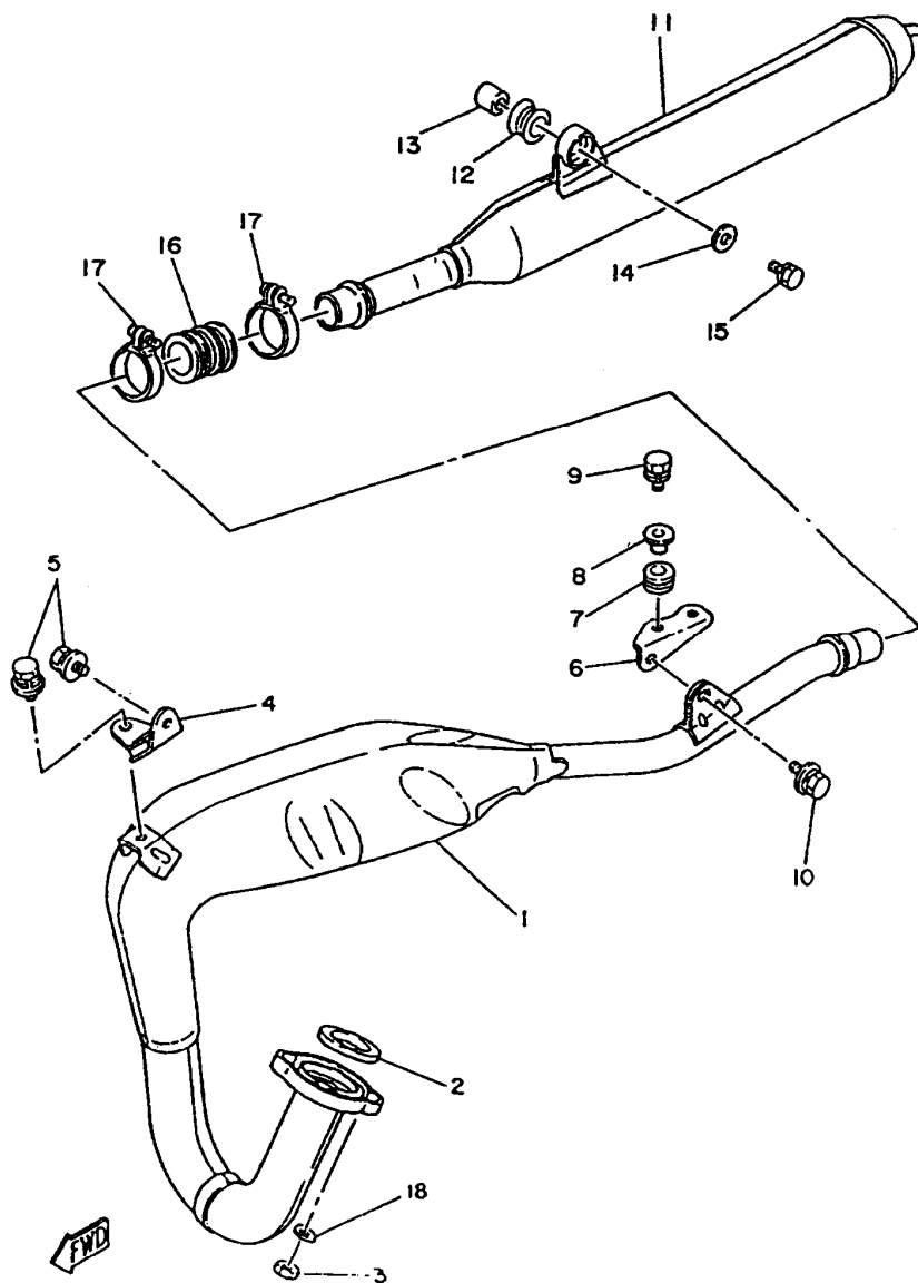
FIG. 13 - ESCAPAMENTO
