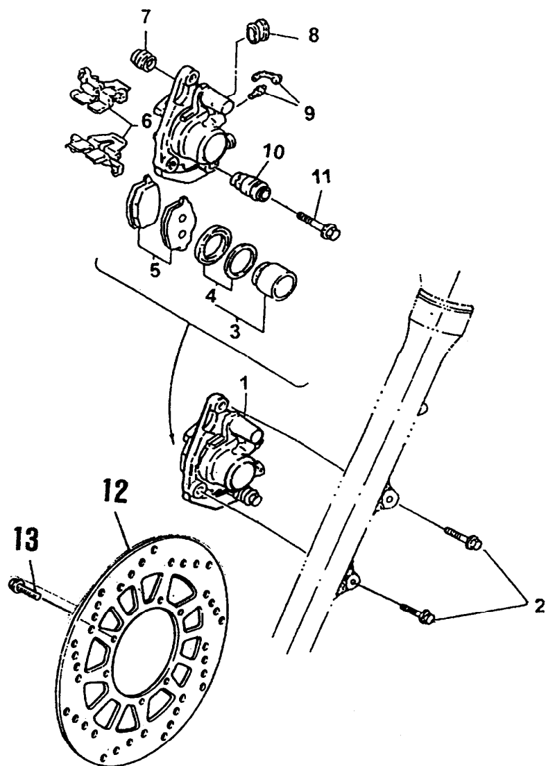
FIG. 35 - DISCO E PINÇA DO FREIO
