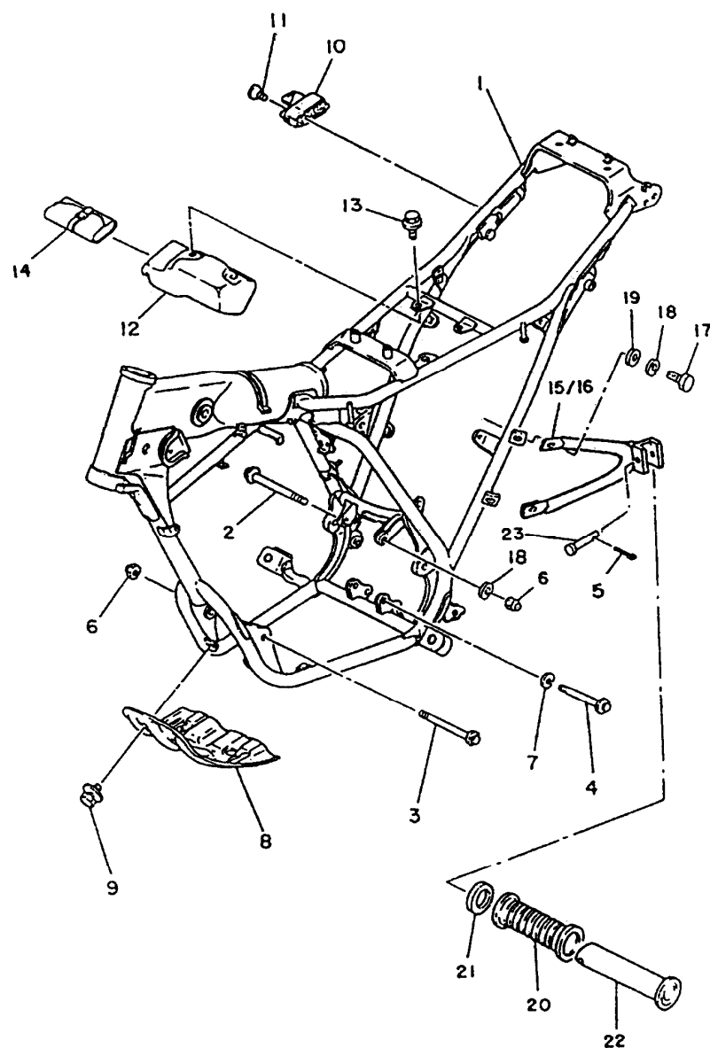
FIG. 16 - CHASSI
