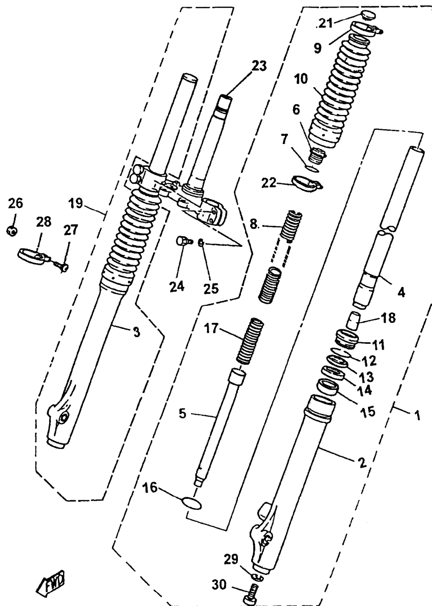
FIG. 21 - GARFO TELESCÓPICO
